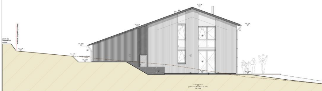
Façade ouest
