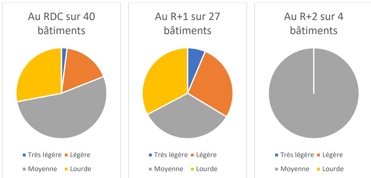
Graphique 4 – Classe d'inertie de constructions en paille en fonction des niveaux (Floissac, 2012)
