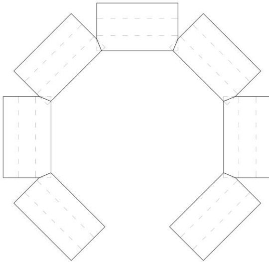
Disposition et dimensions des ballots horizontaux
