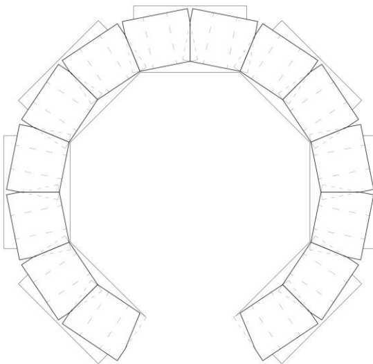
Disposition et dimensions des ballots verticaux
