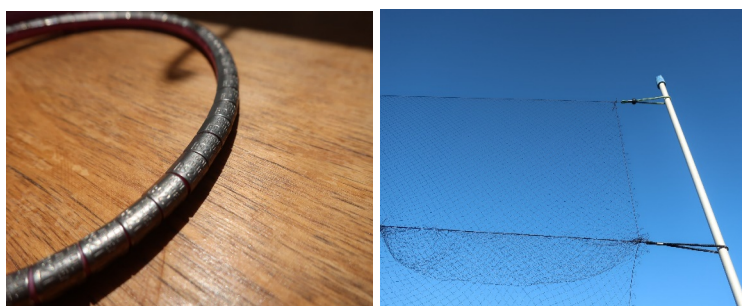
Figure 5 A gauche : photo des bagues en aluminium pour Lanius senator ; A droite photo d'un des filets de capture installés sur Anticythère (Léa Escoutay, 2021)
