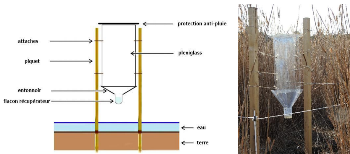
Figure 7: Piège à Polytrap TM
