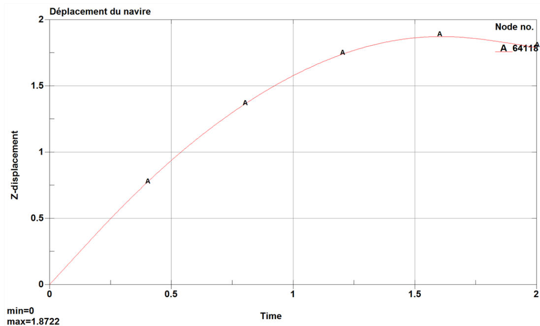
FIGURE 4.1 – Enfouissement maximum du bateau pour le modèle de référence
