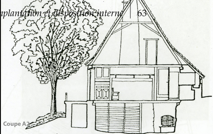
Figure 3.20 - Plans et coupes de la maison saisonnière d'Espargillère et de la ferme de Monceaux-sur-Dordogne
