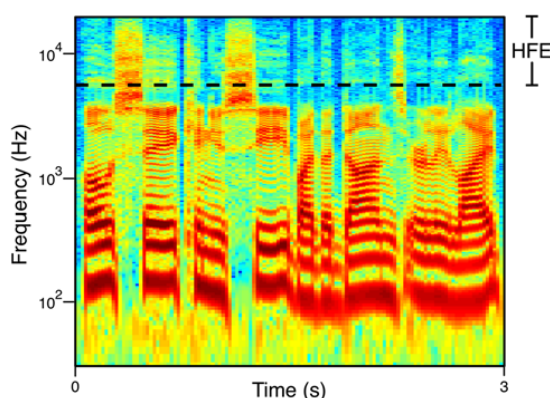
Figure 2 : Spectrogramme de la phrase « Oh say can you see by the dawn's early light » (Monson, Lotto et al., 2014) prononcée par un homme. Sur cette figure la délimitation de la plage des HFE (les bandes d'octaves 8 et 16 kHz) est mise en évidence par une ligne en pointillés.
