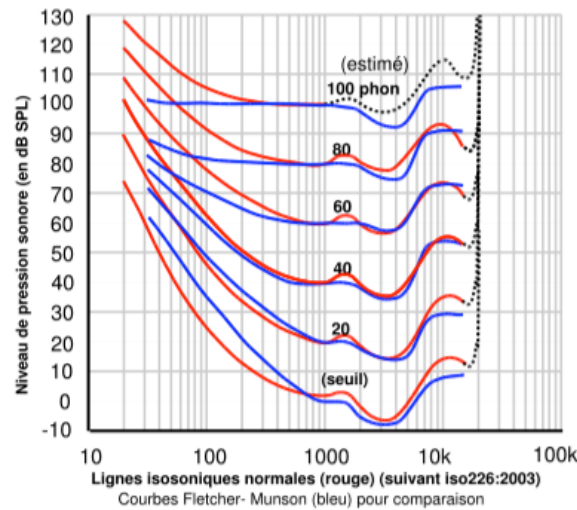
Figure 1 : Lignes isosoniques normales (Vallot, 2019)
