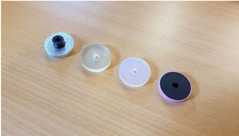
FIGURE 3.20 – Les différentes roues testée pour l’entraînement, en partant de la gauche : aluminium brossé, polyuréthane lisse, silicone légèrement granuleux et PLA avec revêtement en silicone
