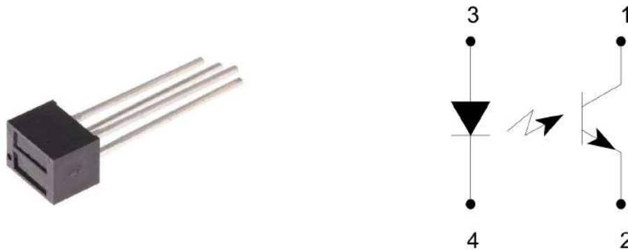
FIGURE 7.2 – Boîtier du capteur avec un schéma des composants présents
