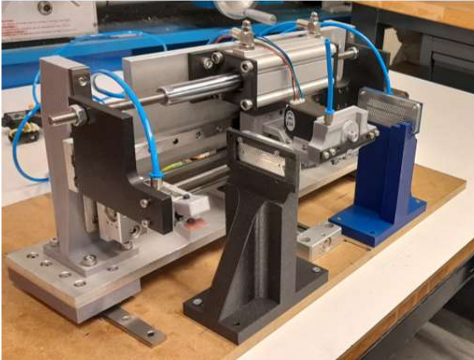
FIGURE 1.9 – Première conception de la machine à tuber
