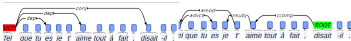
Fig. 82 — Prédiction et correction de PA-1
