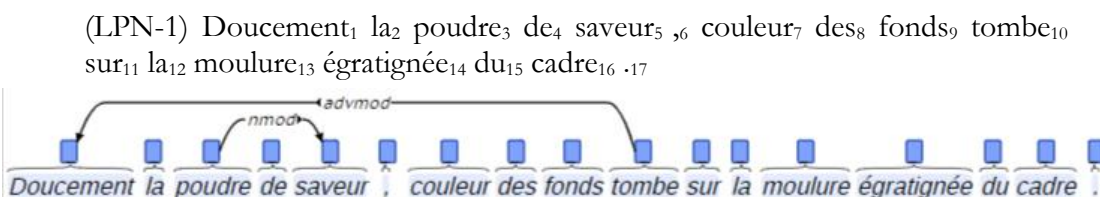
Fig. 20 — Dépendances de LPN-1 de longueur 9 et 2
