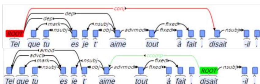
Fig. 78 — Prédiction et correction de PA-1
