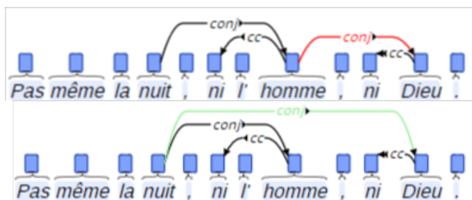
Fig. 28 — Prédiction et correction de G-7
