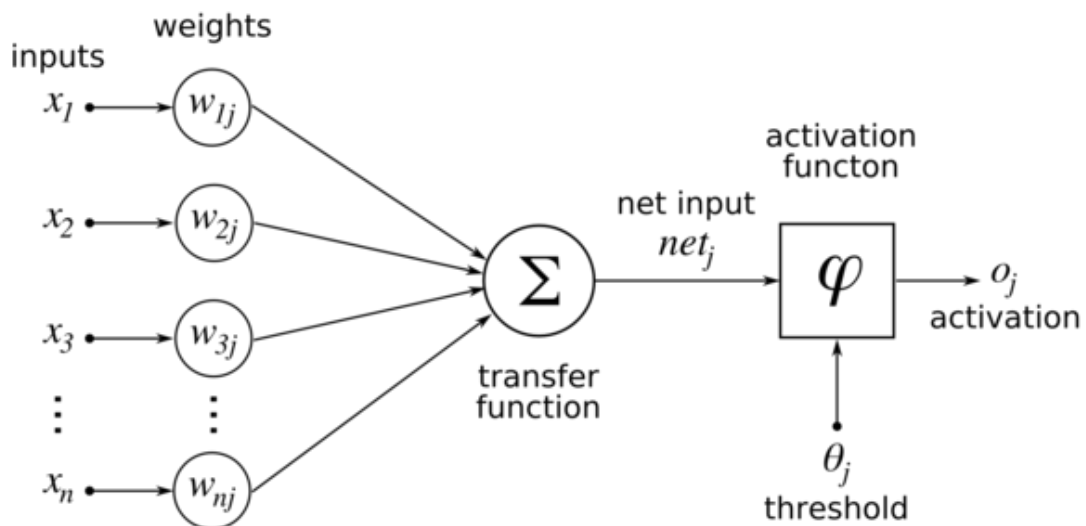
Fig. 1 — Représentation graphique d'un neurone artificiel (Rohrmanstorfer et al. , 2021)
