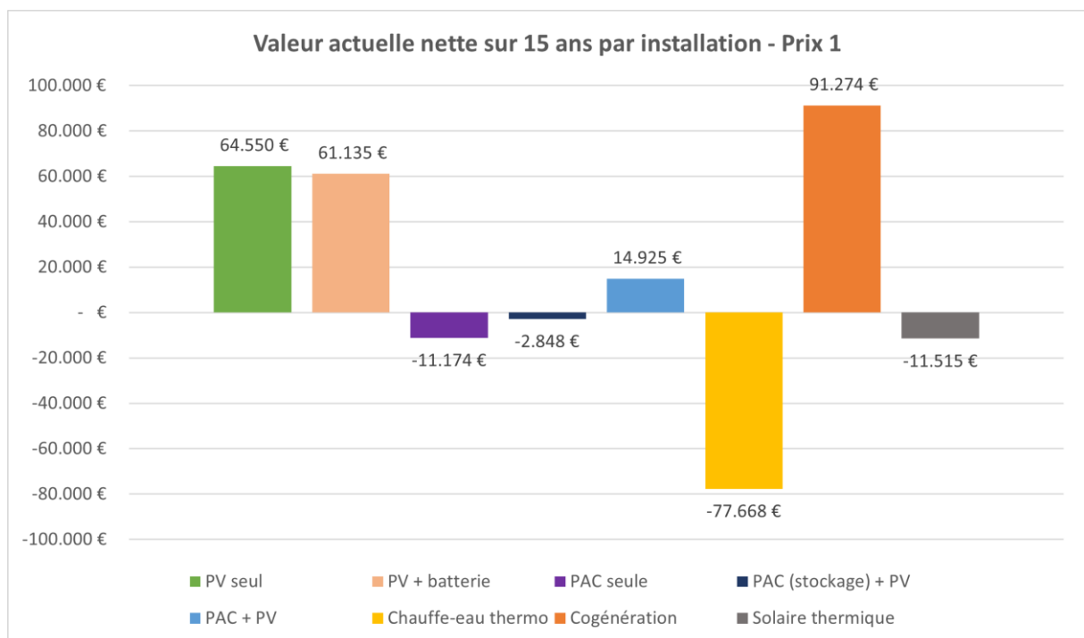
Figure 65 - Comparaison de la valeur actuelle nette sur 15 ans par installation - Prix 1
