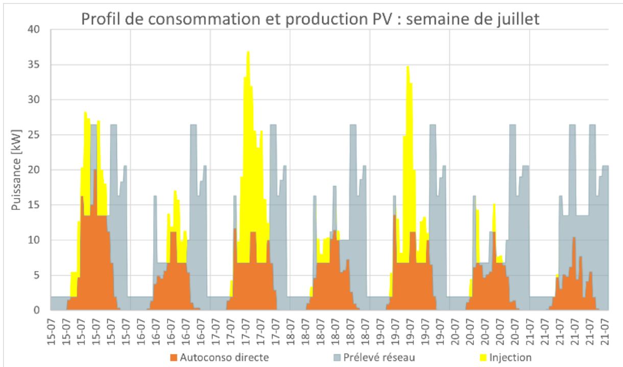
Figure 45 - - Exemple de la consommation et production PV d'une semaine de juillet
