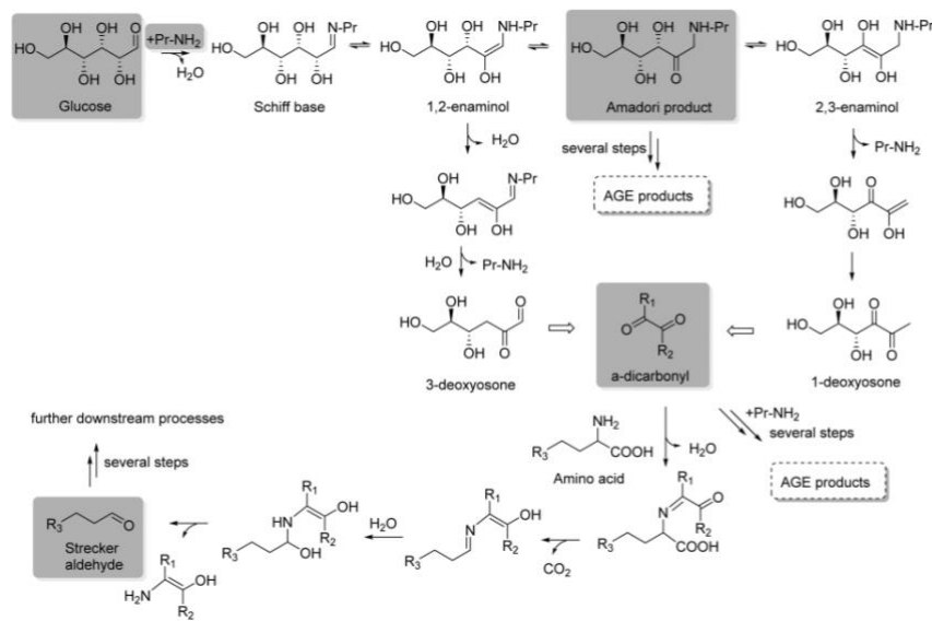
Figure 18 : Schéma simplifié de la réaction de Maillard (Lund et Ray, 2017).
