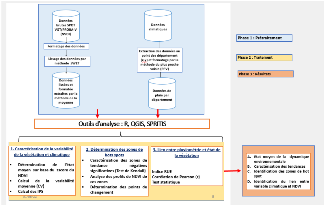
FIGURE 5 Algorithme des grandes opérations de la méthodologie
