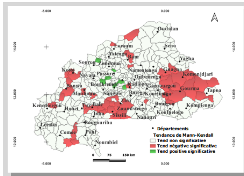
FIGURE 12 : Tendances du NDVI entre 1999 et 2020 au Burkina Faso [seuil de 5%]
