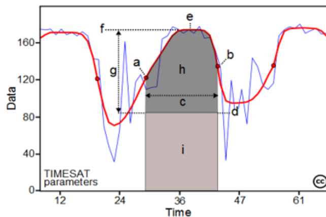
(g)- SOS (b)- EOS (c)- Durée de la saison (d)- Valeur de Base (en unité d'indice de végétation) (e)- Milieu de la saison (f)- Maximum de l'indice de végétation (g)- Amplitude de l'indice de végétation (h)- Petite intégrale (h et i)- Grande intégrale.
