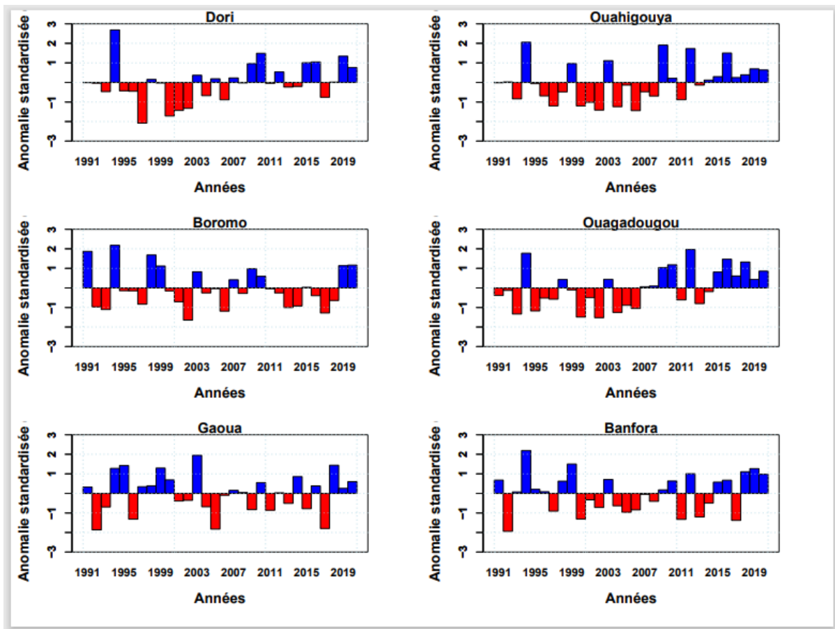
FIGURE 7 Variabilité pluviométrique interannuelle au niveau quelques stations suivant le gradient Nord-Sud (barre rouge : année sèche et barre bleue : année humide)
