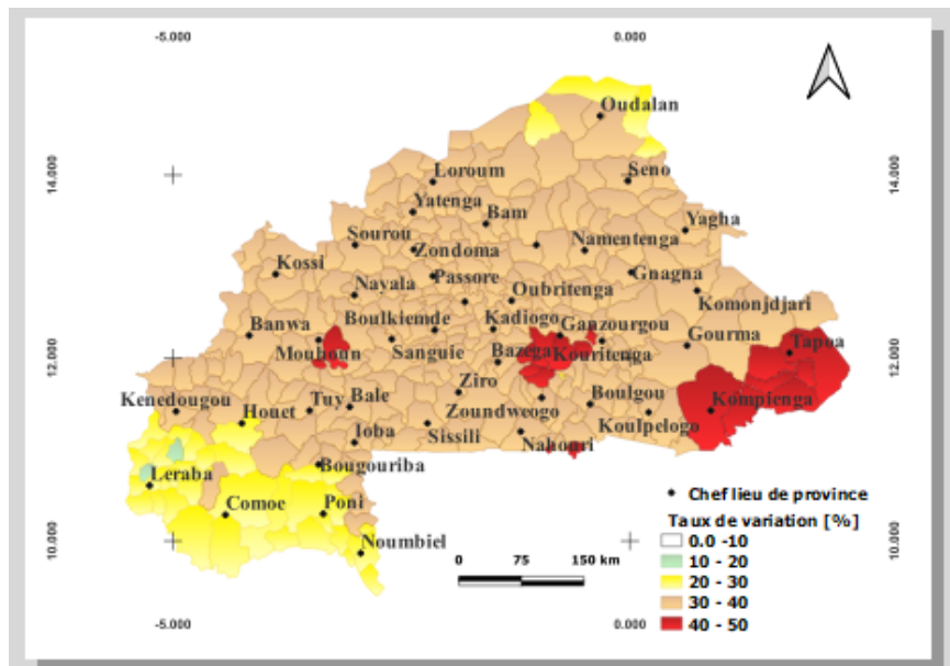
FIGURE 11 Variation moyenne intra-annuelle du NDVI au Burkina Faso de 1999 à 2020
