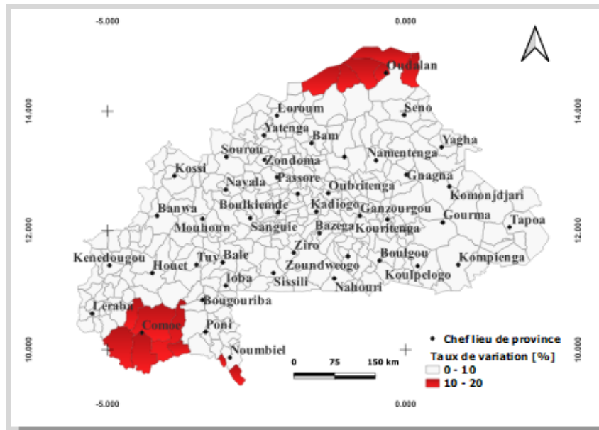
FIGURE 10 Variation moyenne annuelle du NDVI au Burkina Faso de 1999 à 2020
