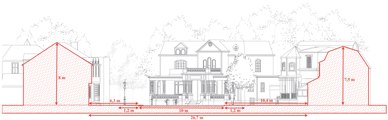
Figure 40 : Coupe relation largeur route/hauteur maison dans Wisteria Lane .
