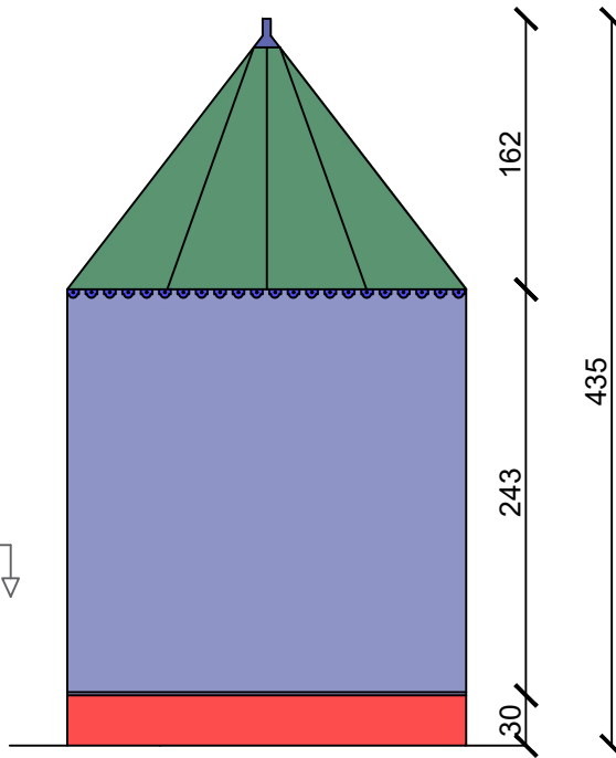
Elév. arrière
