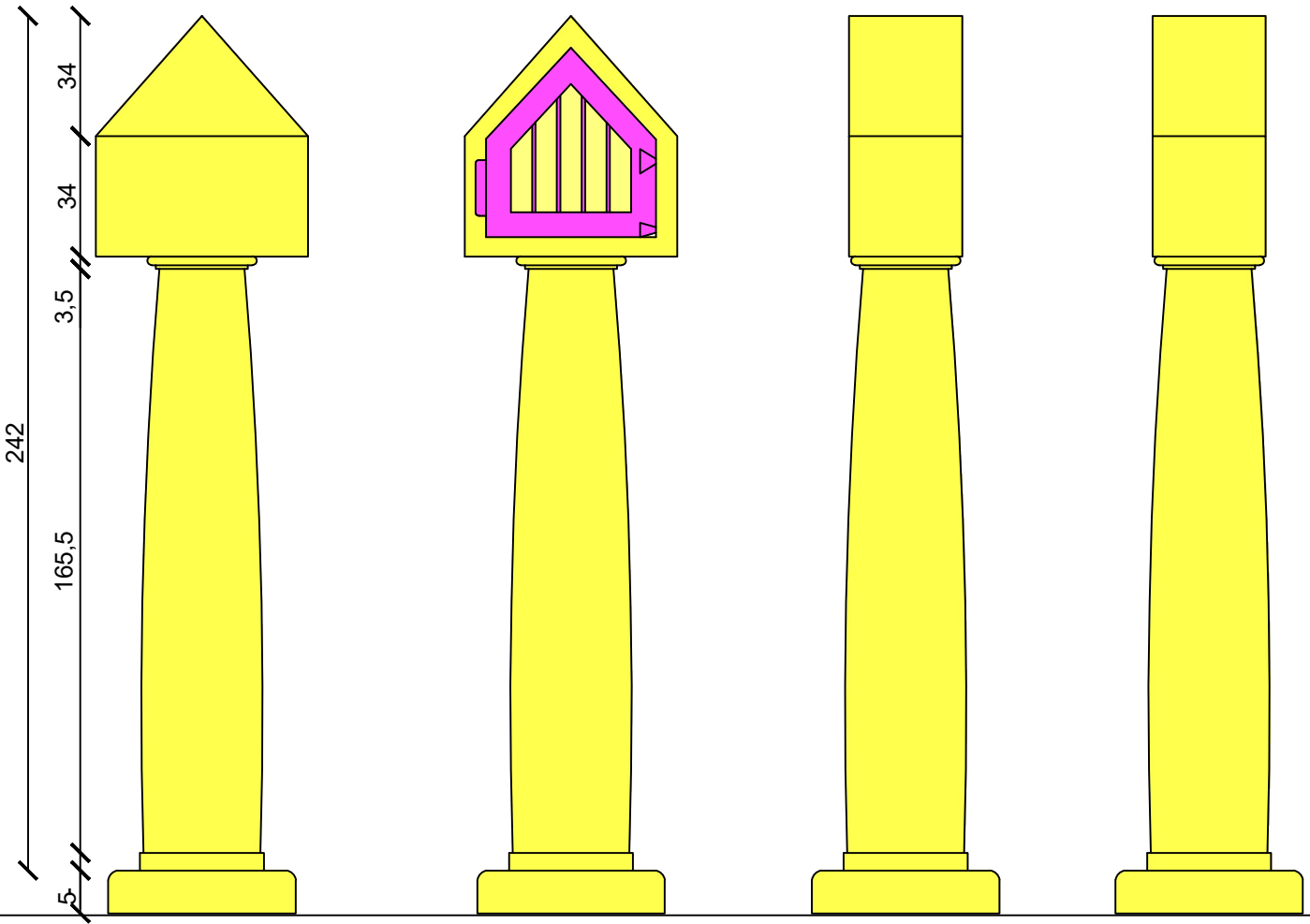
Elév. droite
