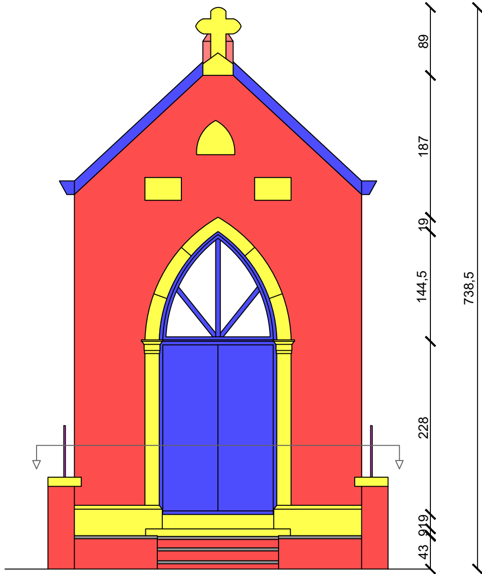
Elév.avant
