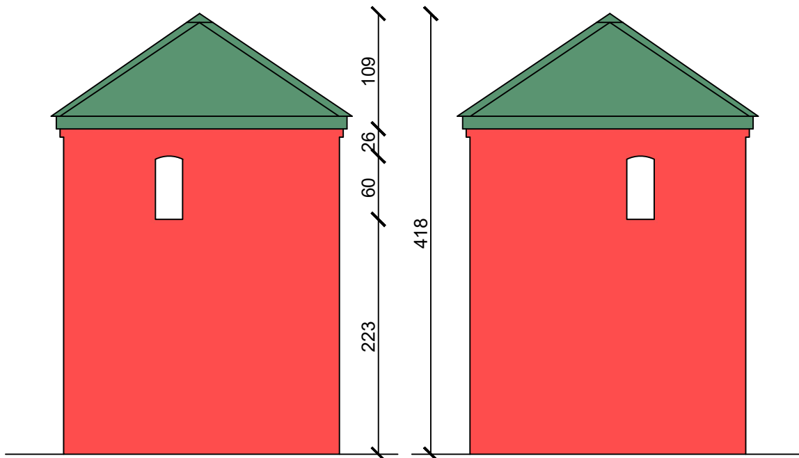
Elév. droite
