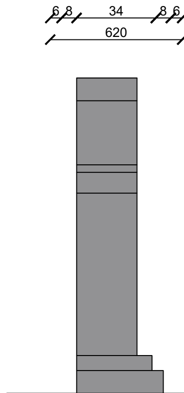
Elév. arrière
