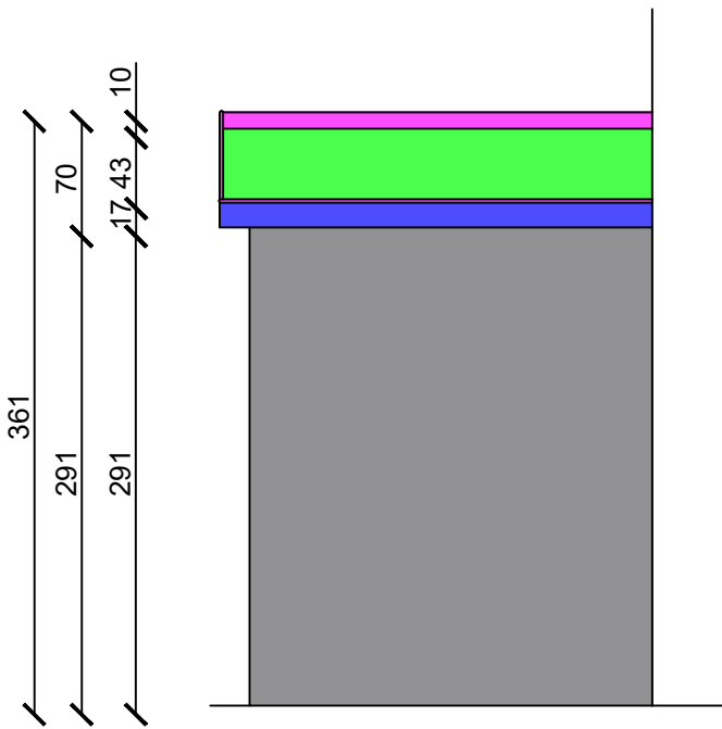
Elév. droite
