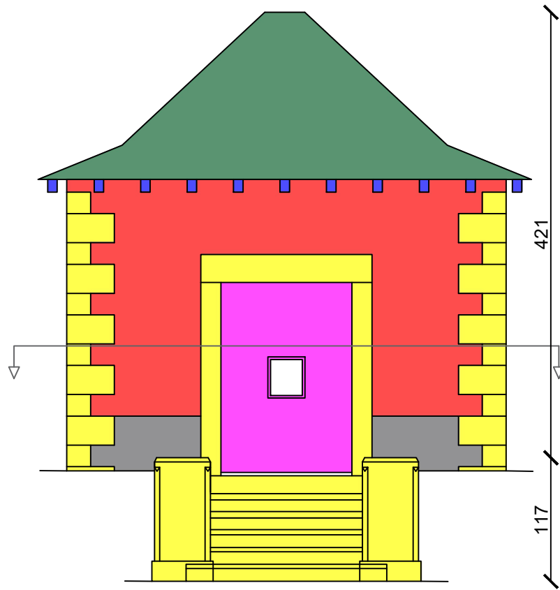
Elév. avant
