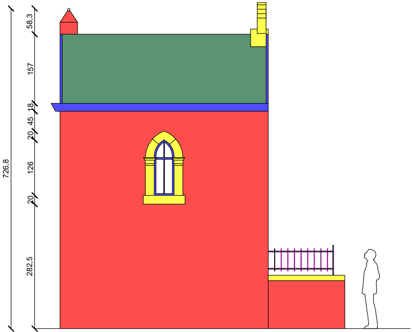
Elév.gauche
