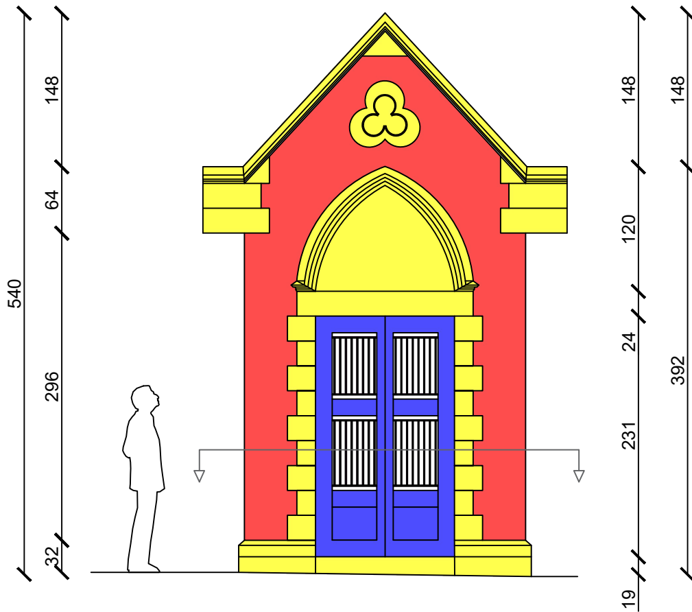
Elév. avant
