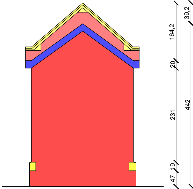
Elév. arrière
