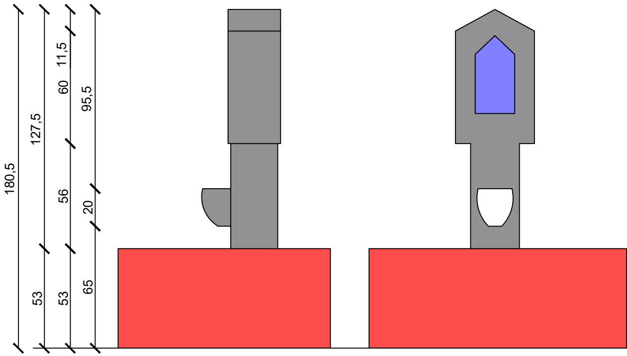
Elév. droite
