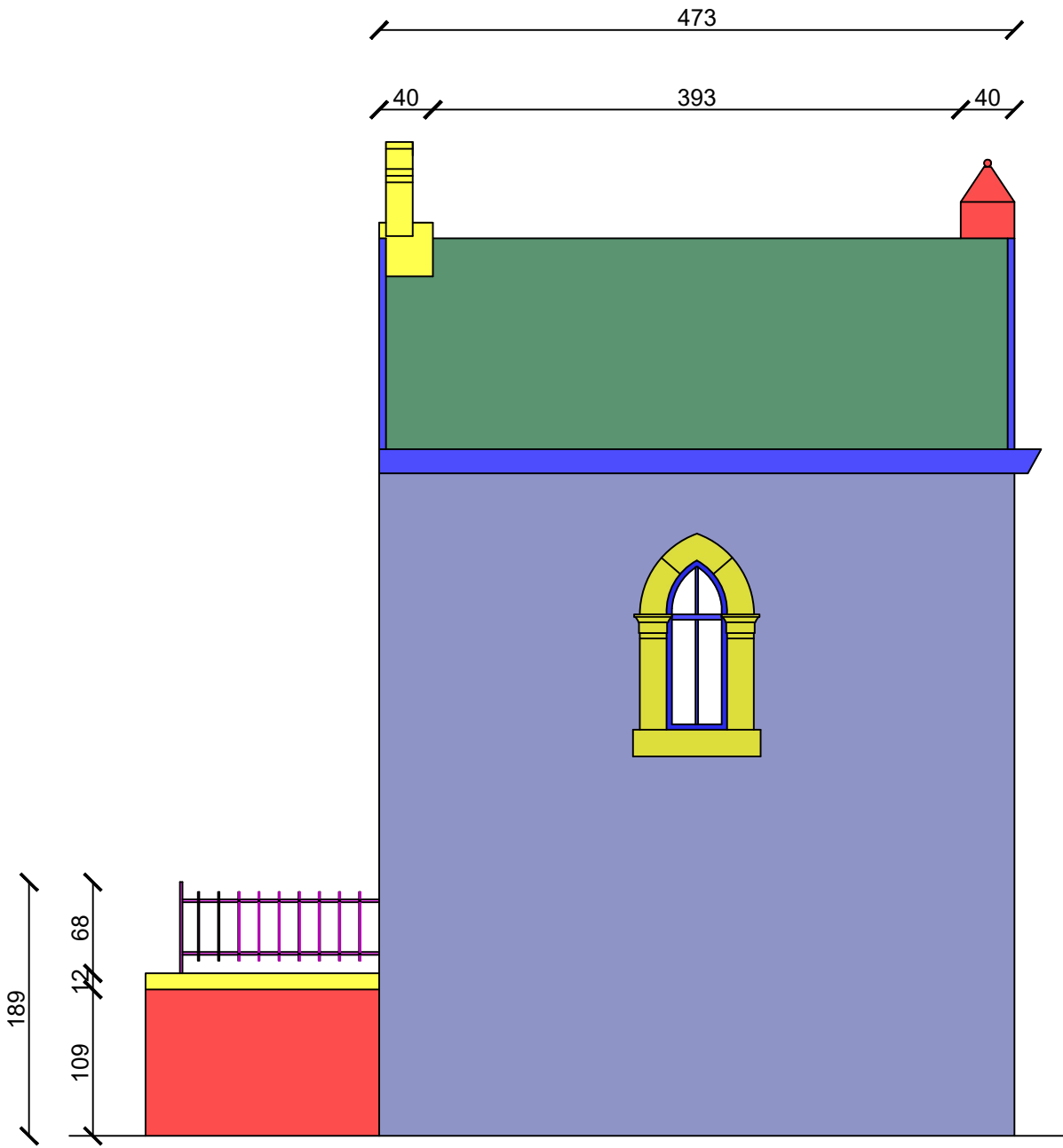
Elév.droite
