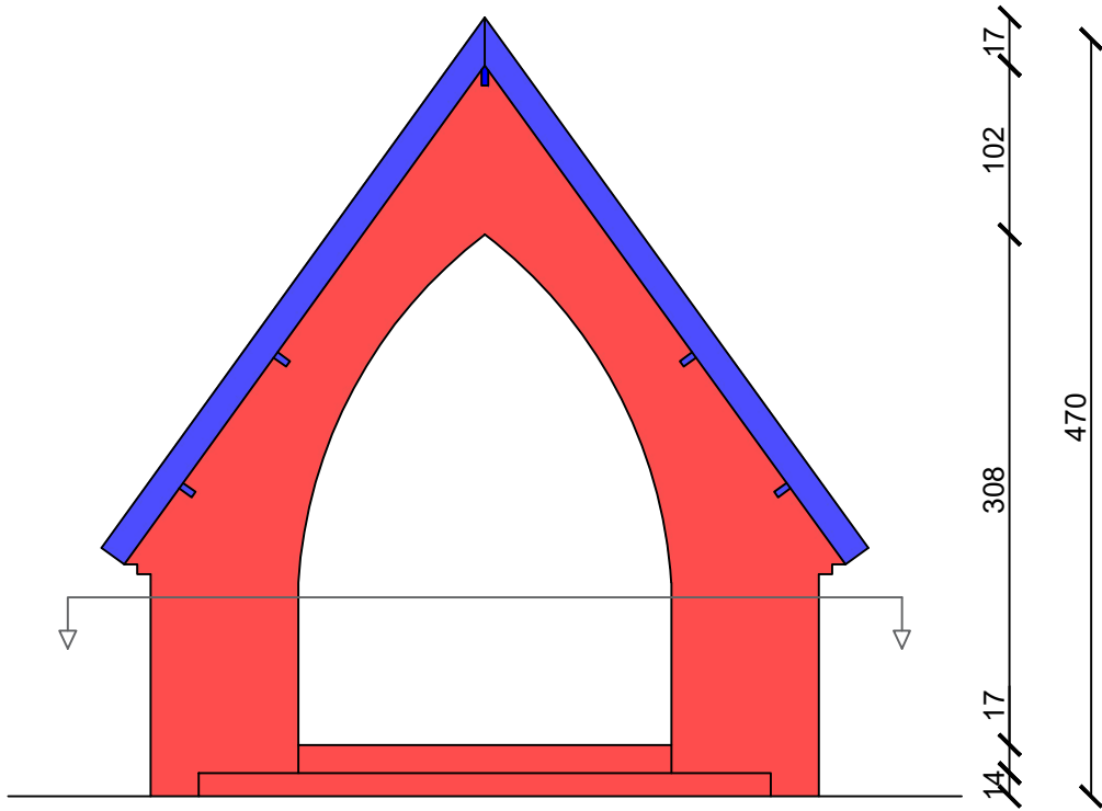
Elév. avant
