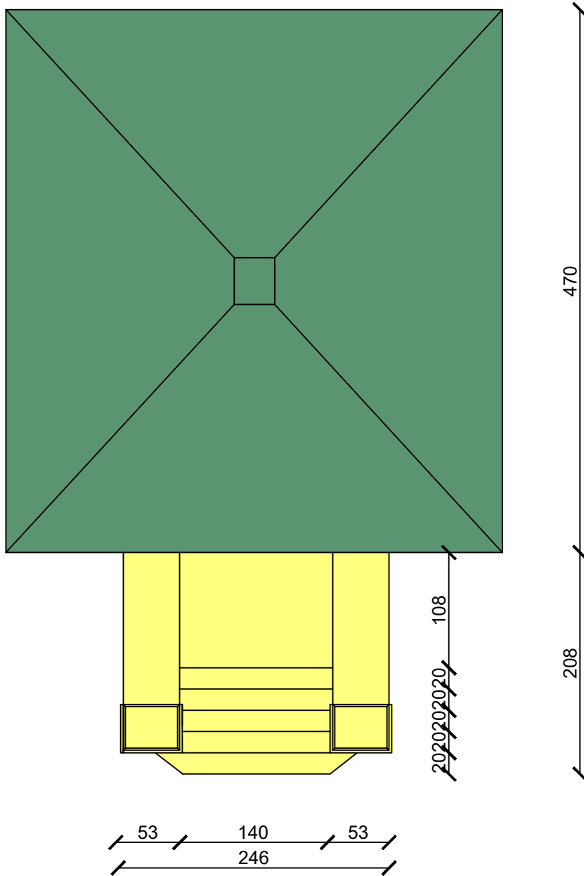
Plan toiture
