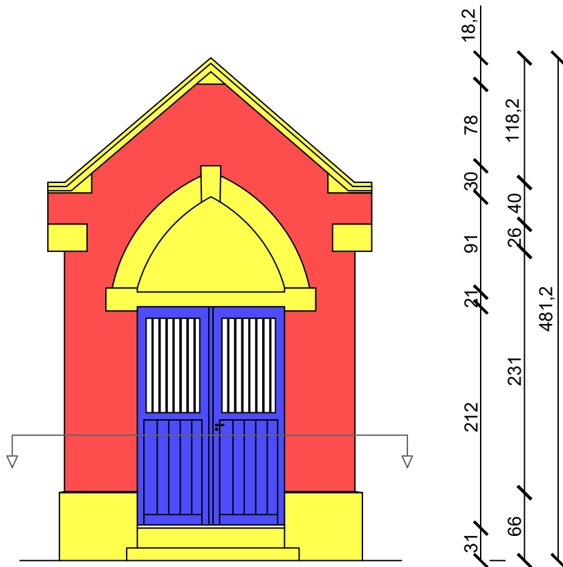
Elév. avant
