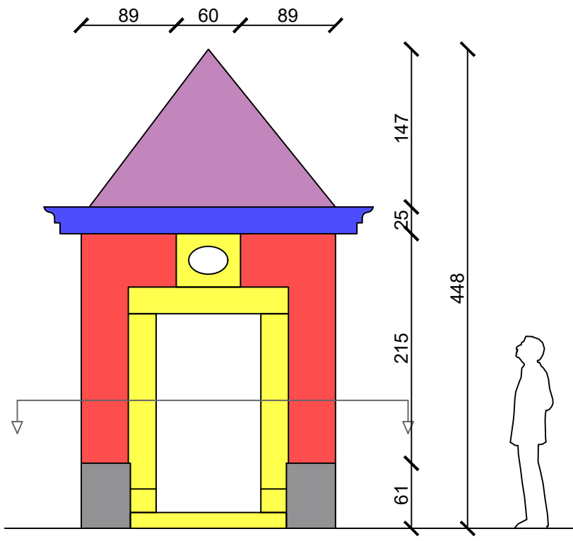
Elév. avant
