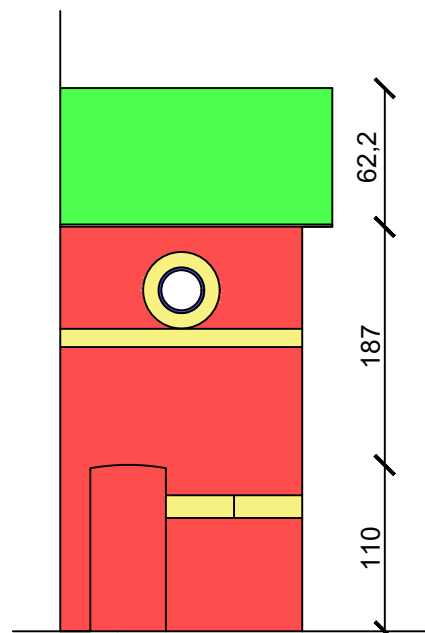
Elév.gauche
