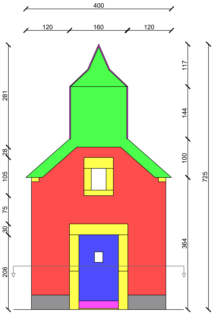
Elév.avant
