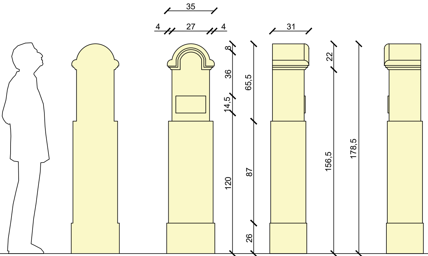
Elév. droite
