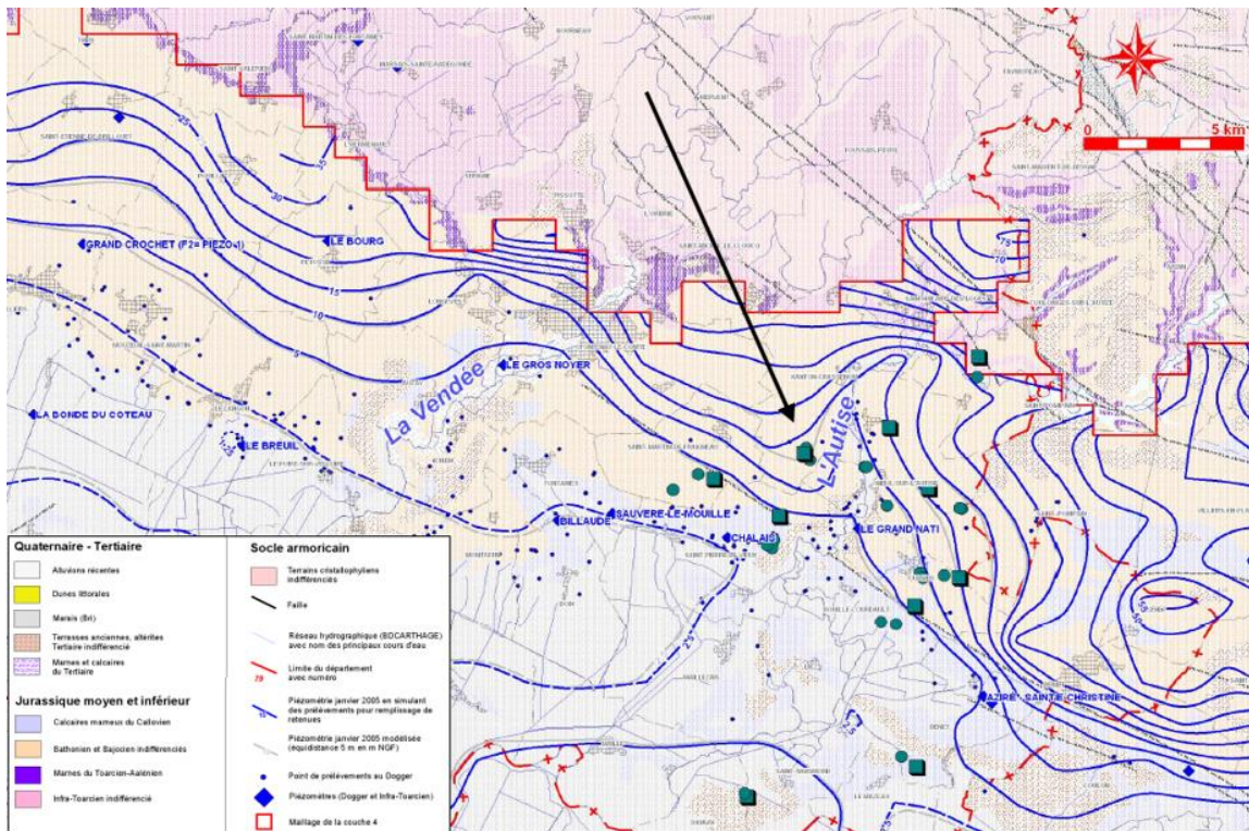
Figure 65: Comparaison des niveaux piézométriques de la nappe du Dogger de janvier 2005 restitués par le modèle avec et sans pompage hivernaux pour le remplissage de retenues de substitution (Doez et al., 2010)
