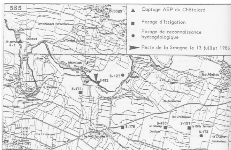
Figure 61: Localisation des forages et de la perte de la Smagne. Communes de Bessay et de St Jean-de-Beigné – Echelle 1/25000 ème (Roy, 1987).
