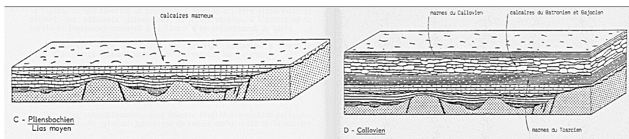
Figure 12: Blocs diagrammes figurant l'évolution de la plaine de Vendée depuis le Jurassique inférieur. A gauche : le Lias moyen. A droite : le Callovien (Roy, 1987). L'orientation Nord Est pointe à droite des figures.
