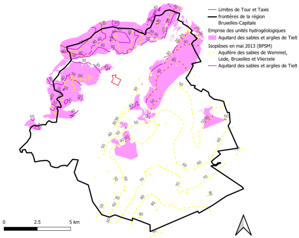
FIGURE 5 – Isopièses de l’aquifère des sables de Wemmel, Lede, Bruxelles et Vlierzele et de l’aquitard des sables et argiles de Tielts.
