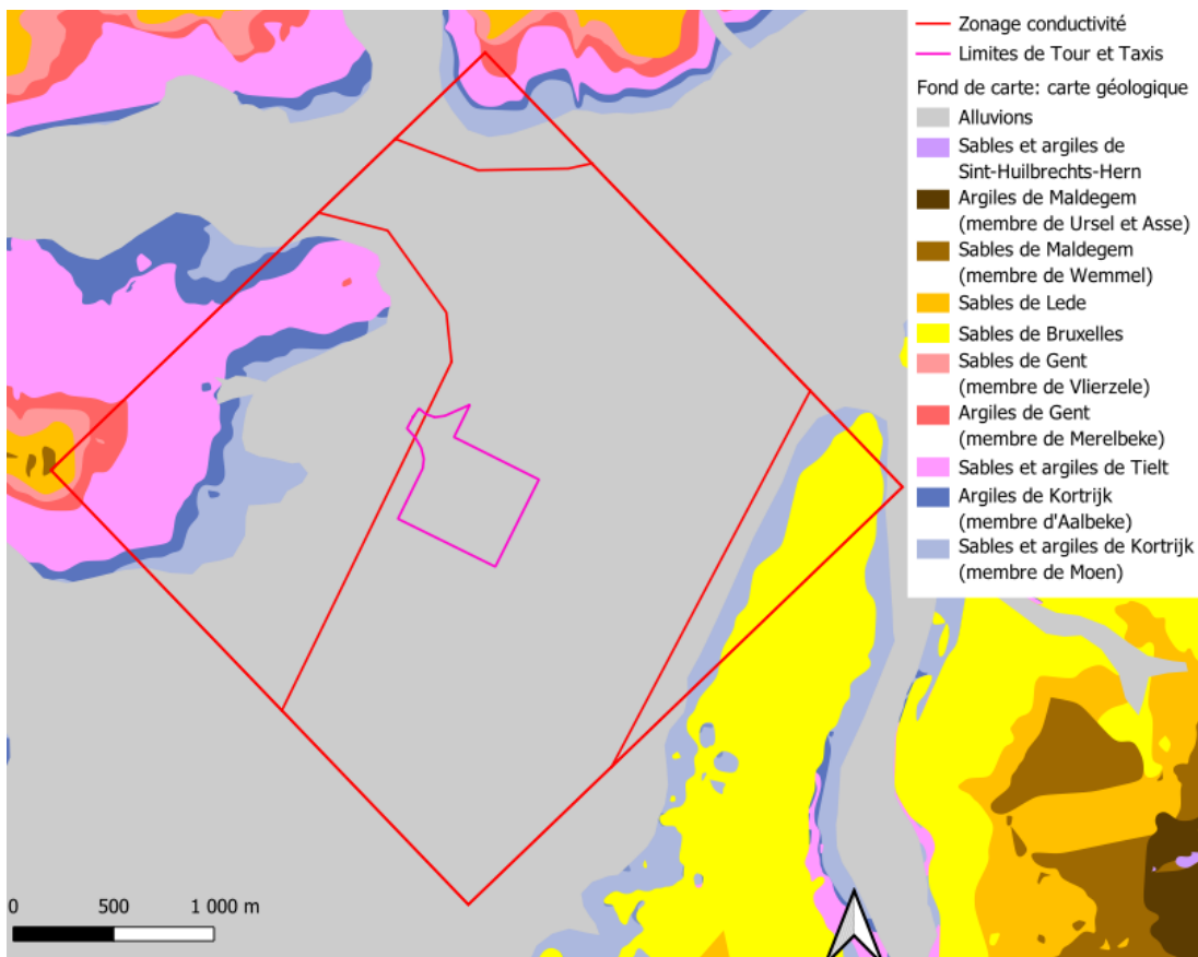
FIGURE 36 – Zonage de la conductivité hydraulique de la première couche du modèle 3D.
