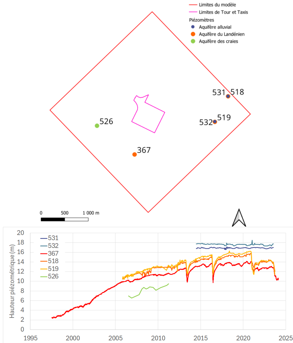
FIGURE 41 – Évolutions piézométriques observées dans la zone du modèle 3D.
