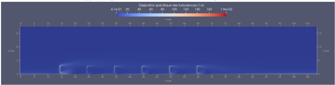
(b) Champ de la dissipation spécifique des turbulences en \text{s}^{-1}
