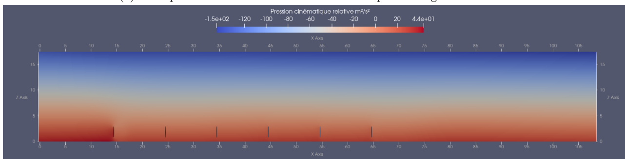
(b) Champ des pressions en \text{m}^2 \text{s}^{-2}
