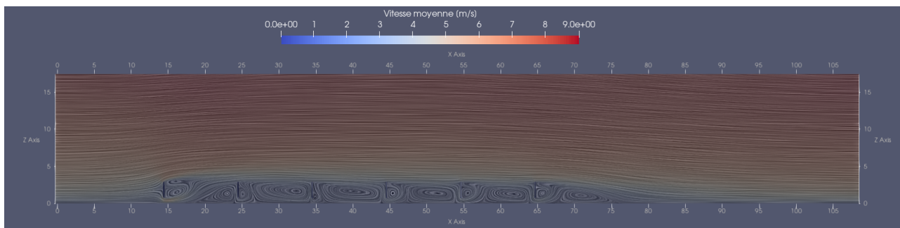
(a) Champ des vitesses en \text{m s}^{-1} . Les tracés indiquent les lignes de courant
