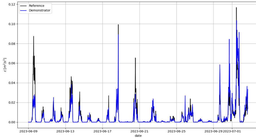
FIGURE 7.2 – Données expérimentales du démonstrateur agrivoltaïque de Valpuseaux pour la dissipation des turbulences \epsilon
