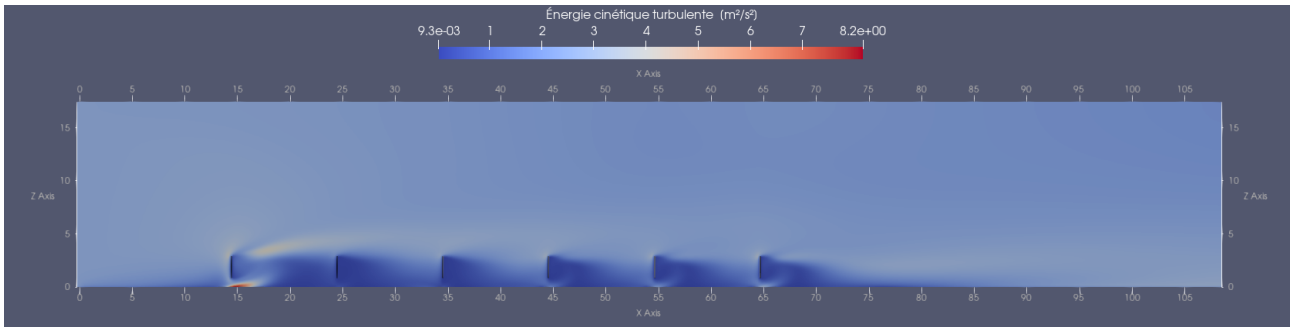
(c) Champ de l'énergie cinétique turbulente en \text{m}^2 \text{s}^{-2} .
