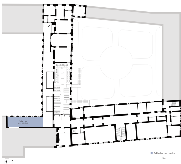
Fig. 49 : Implantation salle des pas perdus au sein du Palais de Justice de Liège
