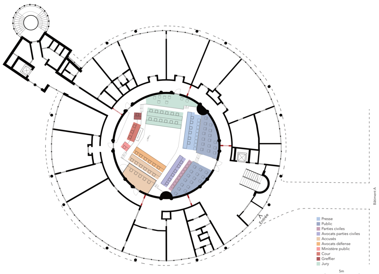
Fig. 19 : Plan de positionnement des acteurs dans la cour d'assises d'Arlon
