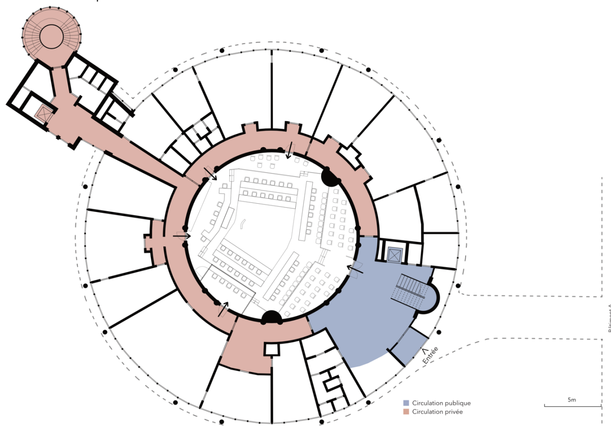
Fig. 18 : Espaces de circulation dans le Palais de Justice d'Arlon
