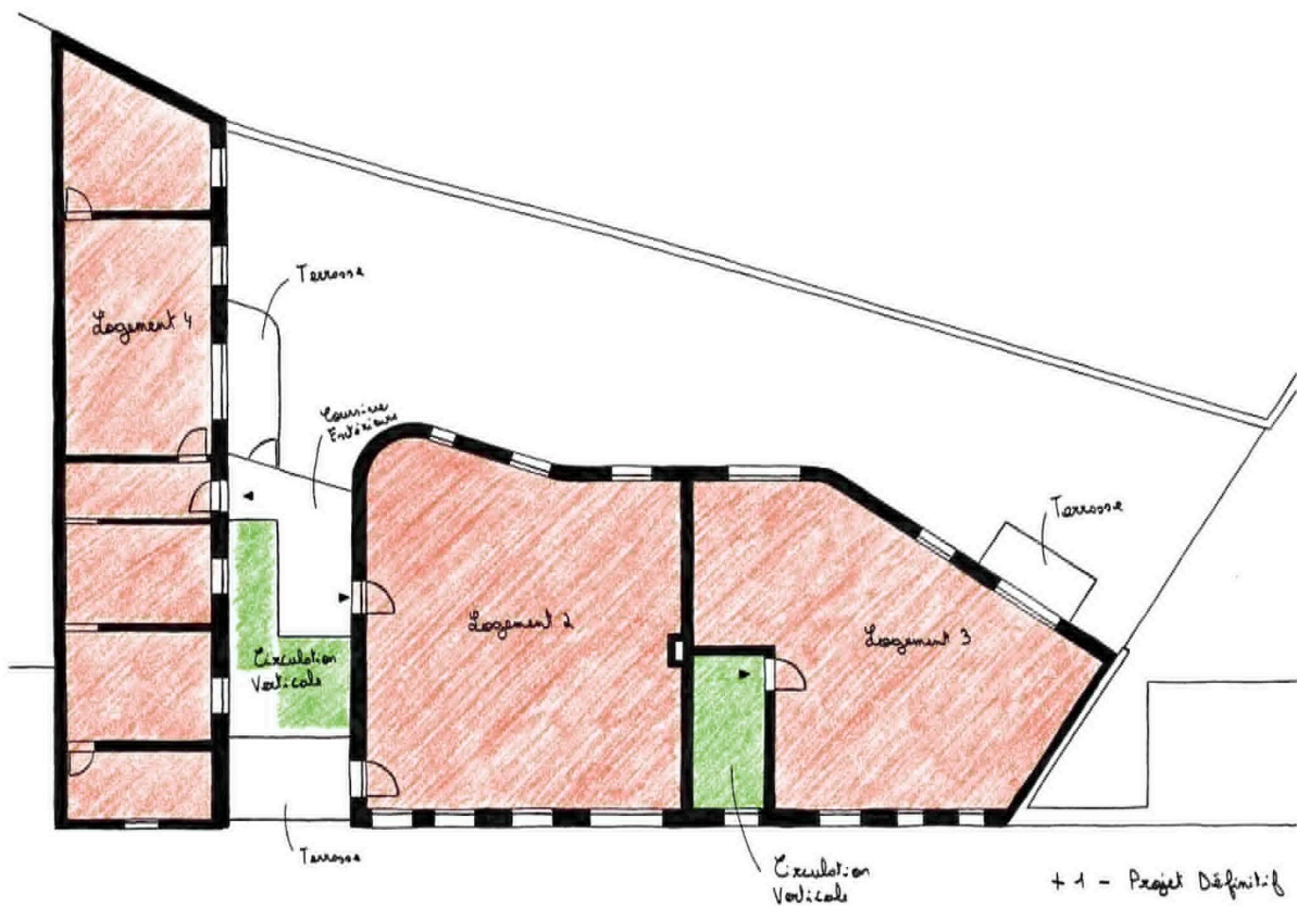
Fig. 16 & 17 : Plan du RDC et du +1 du projet définitif "Gray"
