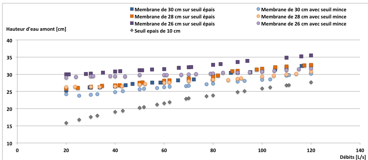
FIGURE E.2 : Hauteurs d'eau retenues par des membranes en Néoprène 34 064 fixés sur des seuils épais ou mince pour des débits variables
