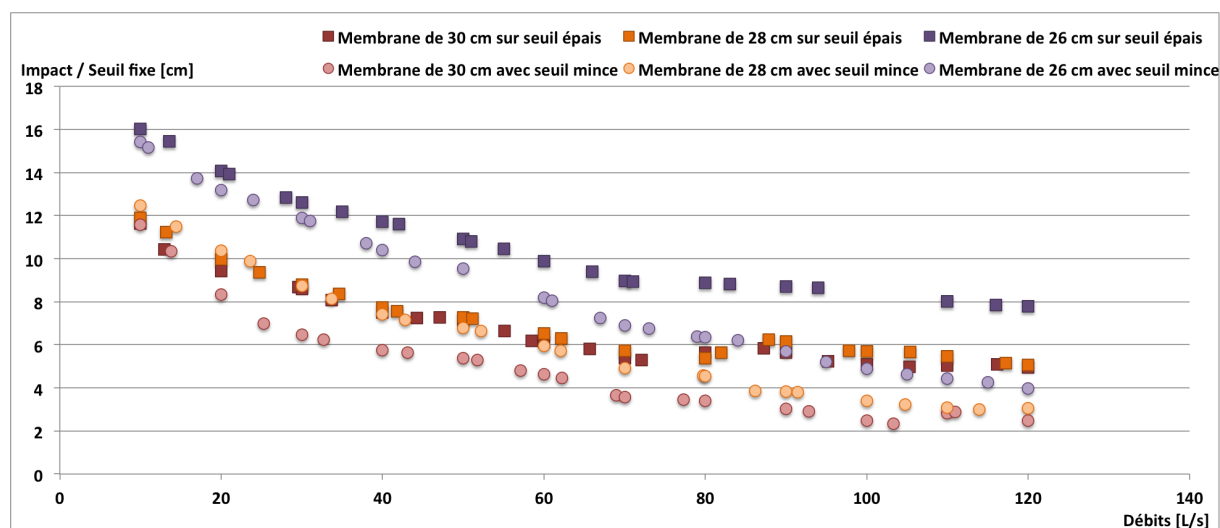
FIGURE 4.30 – Comparaison entre l'impact des membranes sur seuil épais et sur seuil mince avec une limitation des sur-pressions avalles
