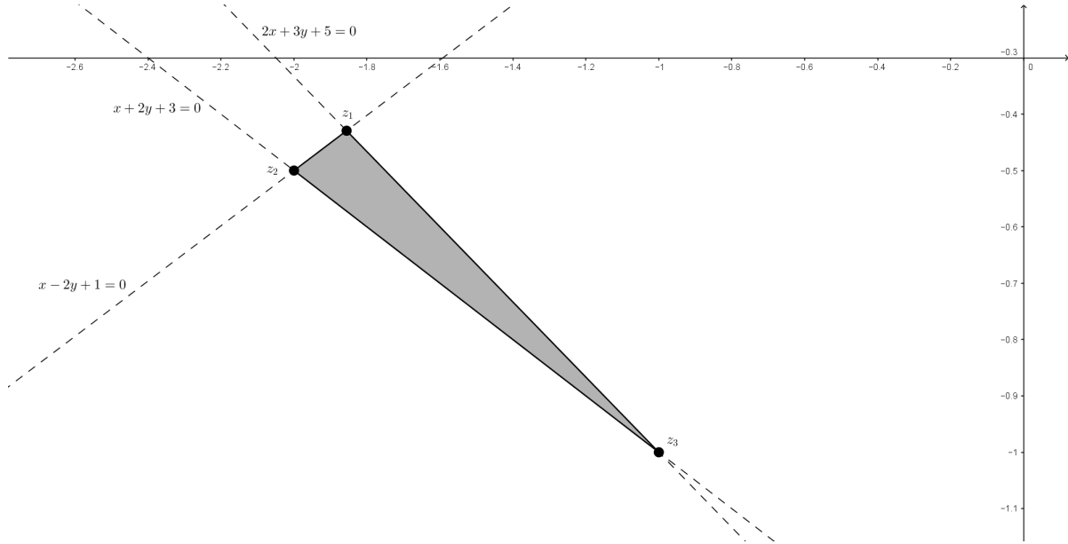
FIGURE 4.1 – Représentation des trois contraintes 2x + 3y + 5 \leq 0 , -x + 2y - 1 \leq 0 et -x - 2y - 3 \leq 0 .
