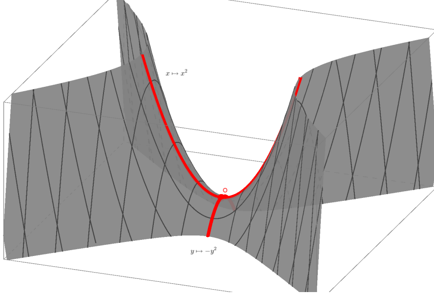
FIGURE 4.2 – Représentation de la fonction F : (x, y) \in \mathbb{R}^2 \mapsto x^2 - y^2 \in \mathbb{R} . On voit facilement que le point (0,0) est un point selle car 0 est minimum de x \mapsto f(x, 0) = x^2 et 0 est maximum de y \mapsto f(0, y) = -y^2 .
