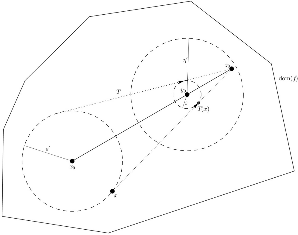
FIGURE 3.1 – Le voisinage B(y_0, \varepsilon) recherché de y_0 est obtenu en effectuant une homothétie T de centre z_0 et de rapport r/(1+r) à l'ensemble B(x_0, \varepsilon') .
