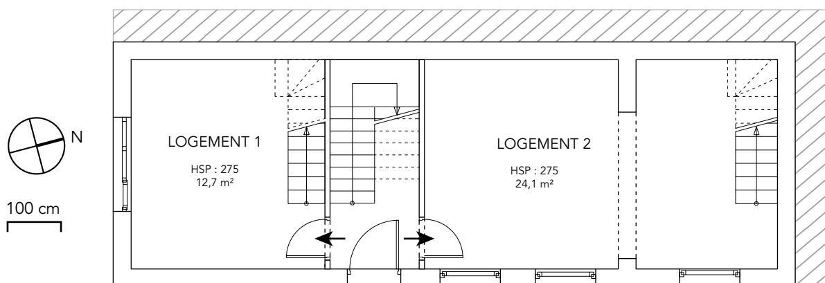
NIVEAU RDC
