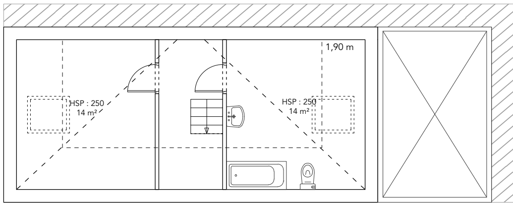
NIVEAU R+3
