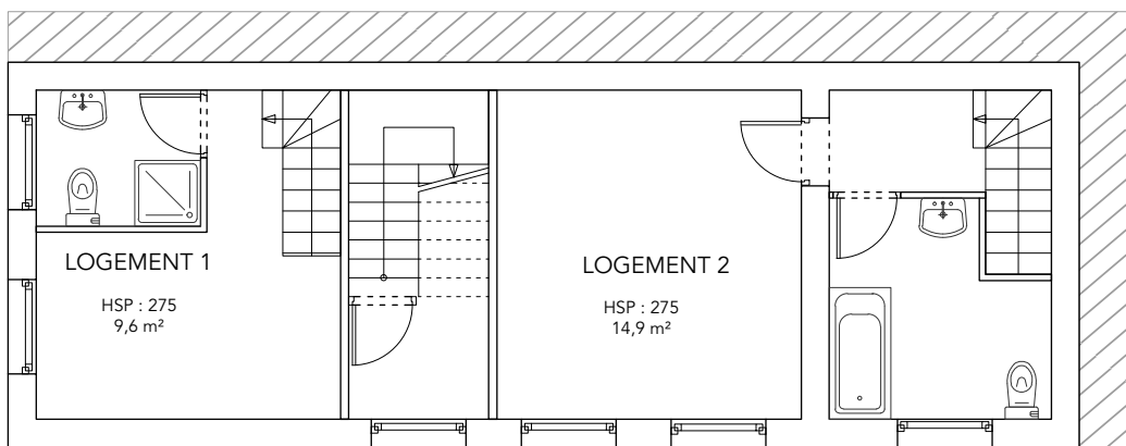
NIVEAU R+1
