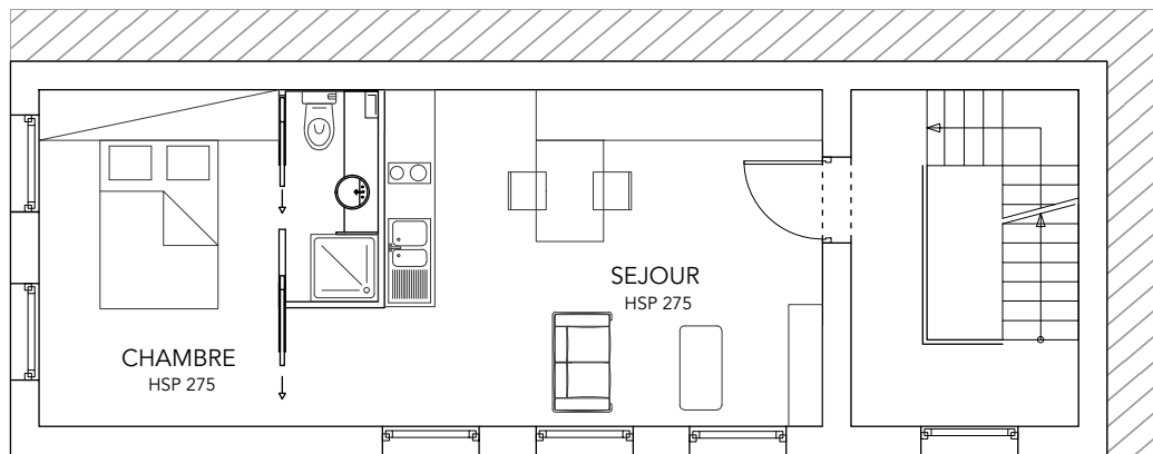
NIVEAU R+1 - LOGEMENT n°2 - 37,2 m²
