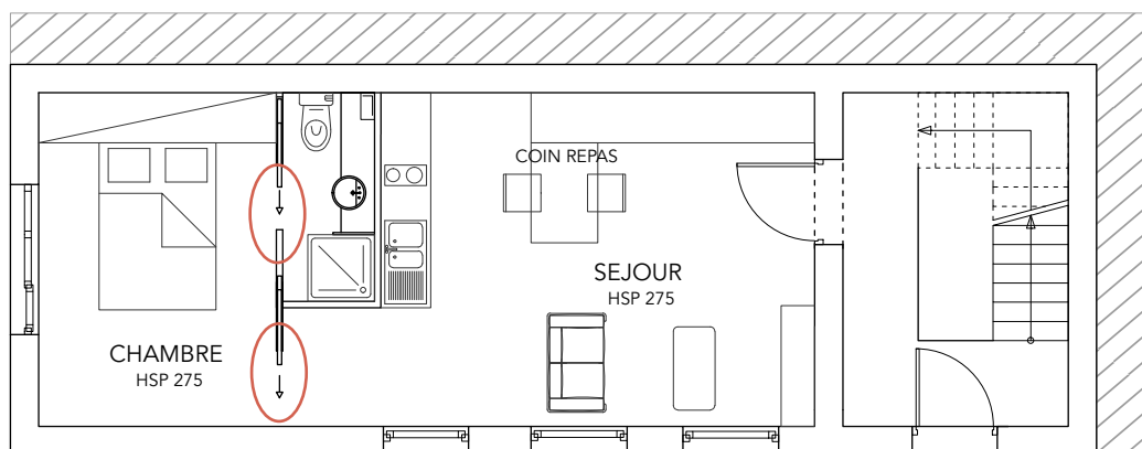
NIVEAU RDC - LOGEMENT n°1 - 37,2 m²
