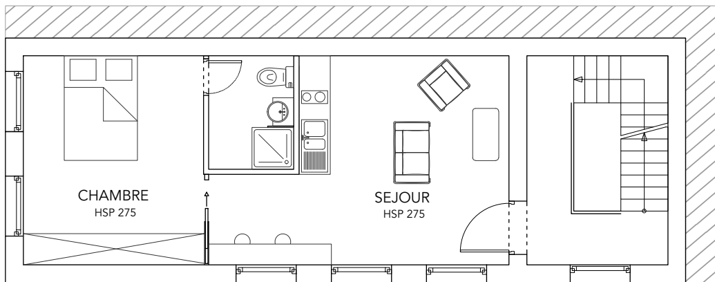
NIVEAU R+1 - LOGEMENT n°2 - 31,2 m 2
