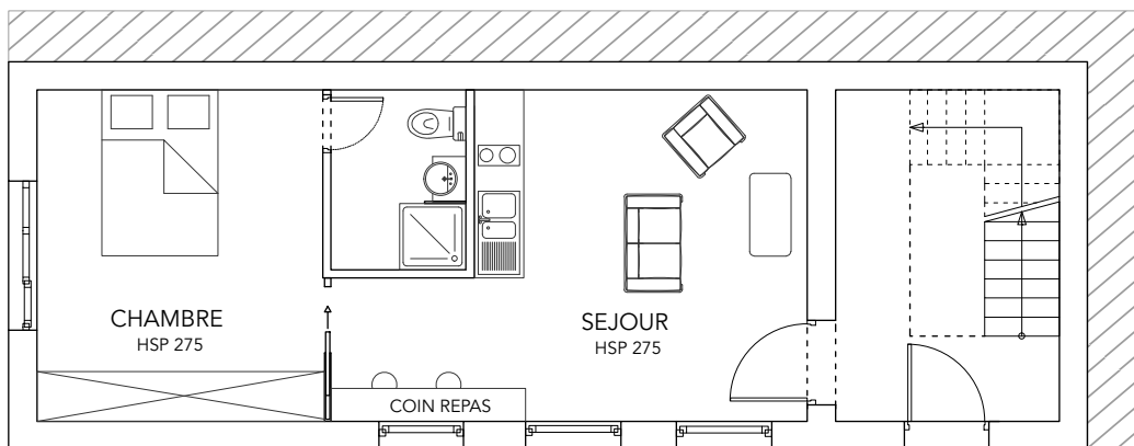
NIVEAU RDC - LOGEMENT n°1 - 31,2 m 2
