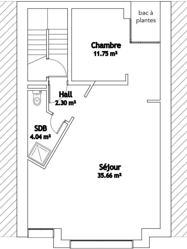
NIVEAU R+1 Logement 1
