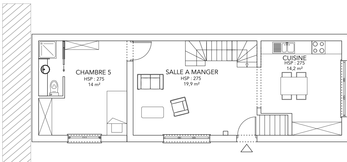
NIVEAU RDC
