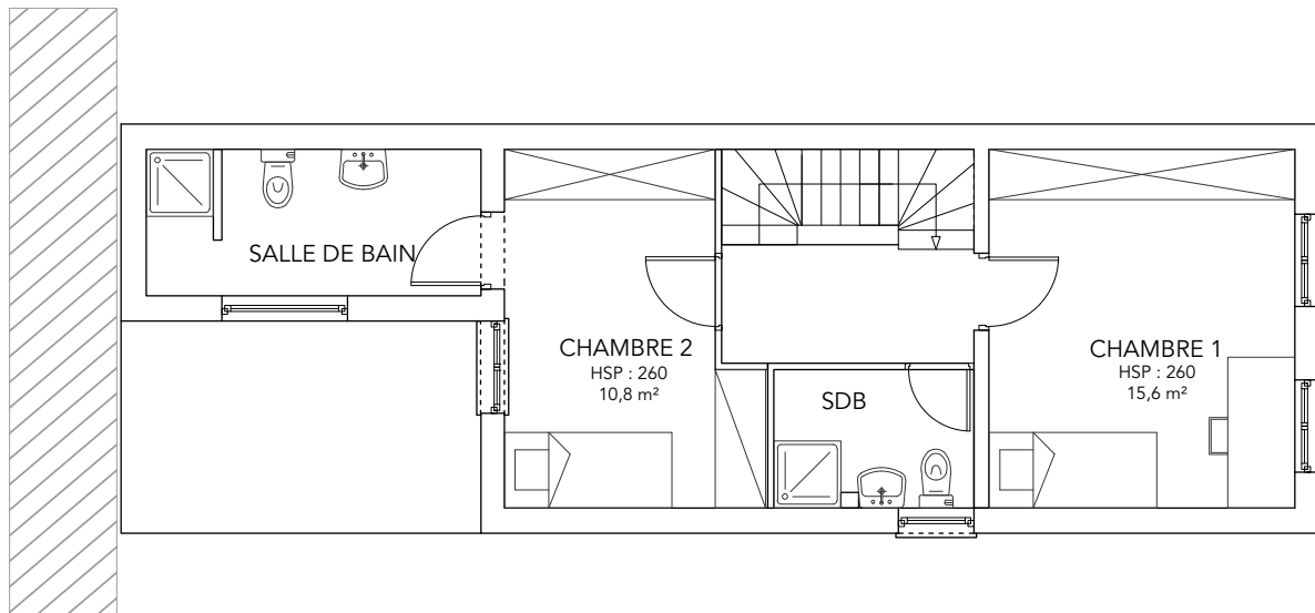
NIVEAU R+1
