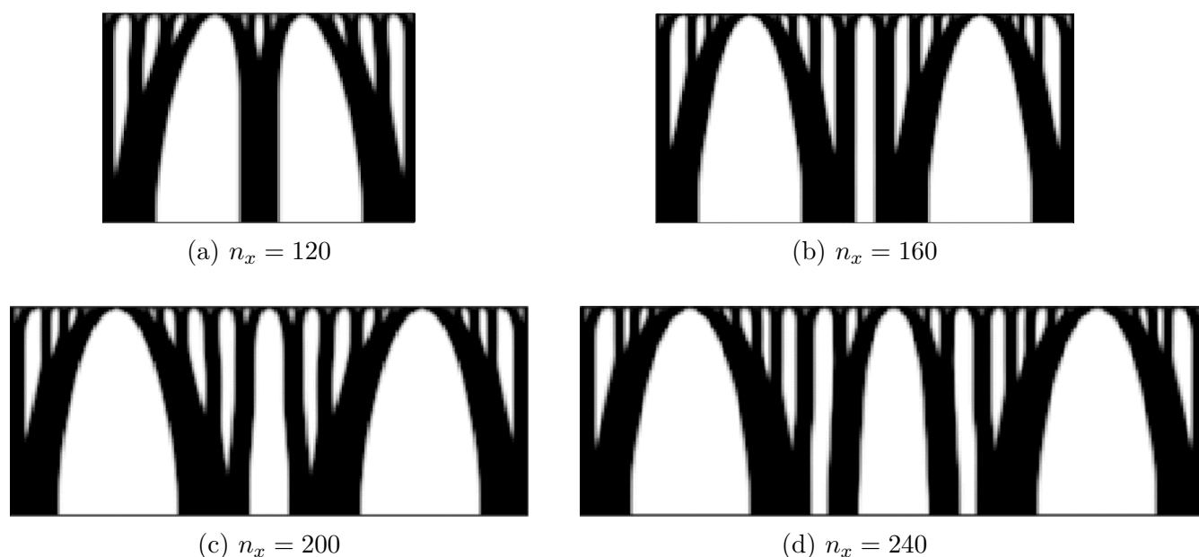
FIGURE 3.9 – Designs obtenus pour le cas 4 en faisant varier le nombre d'éléments n_x , n_y étant maintenu à 80
