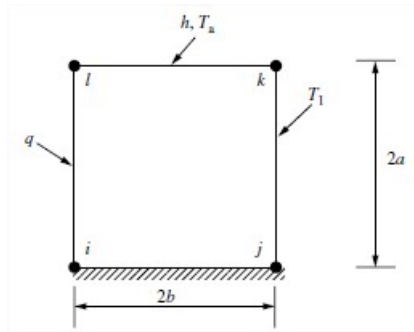
FIGURE 3.3 – Schéma d'un élément rectangulaire pour la méthode des éléments finis ([28])
