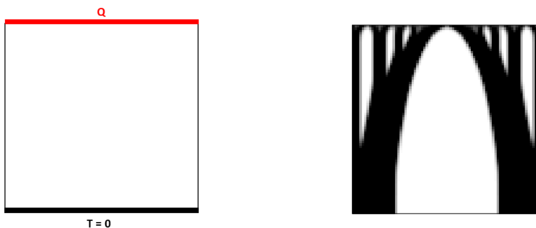
(a) Schéma des conditions aux limites
