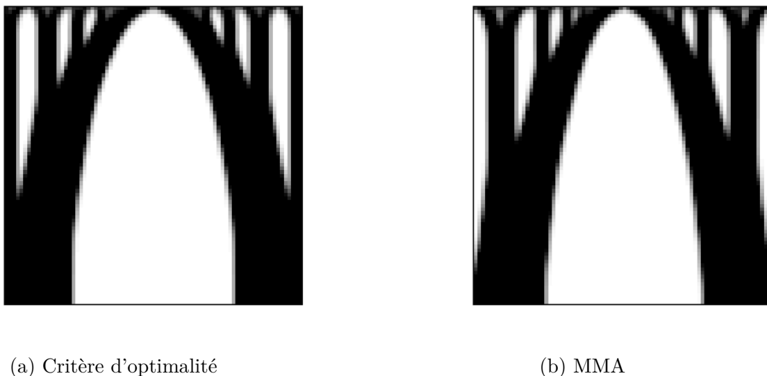
FIGURE 3.11 – Designs obtenus pour le cas 4 avec deux processus d'optimisation différents
