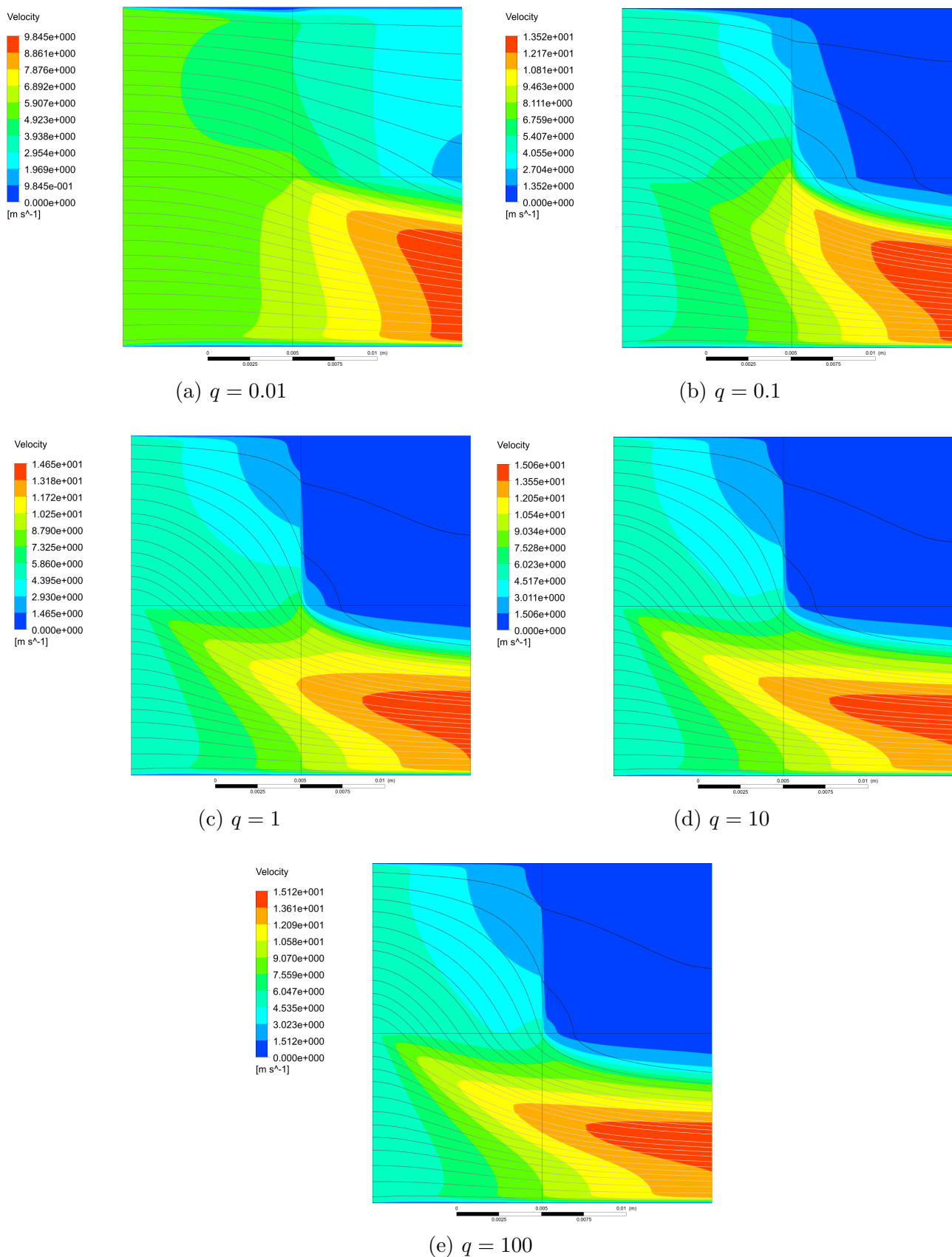
FIGURE 4.13 – Répartition de la vitesse et lignes de courant pour différents paramètres de pénalisation q dans le cas 2x2 avec le vecteur de variable de conception correspondant à la Fig.4.11c
