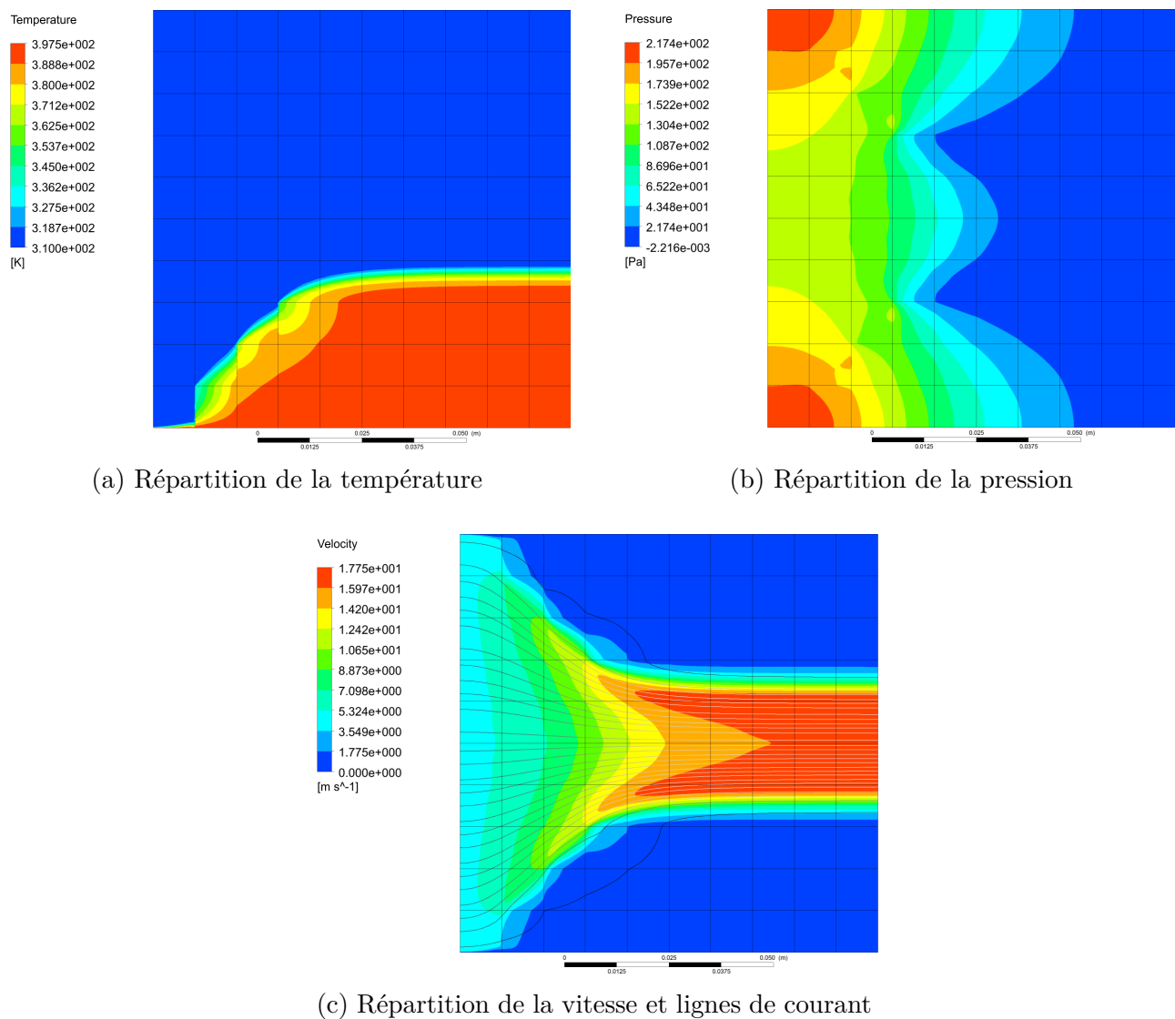
FIGURE 4.16 – Cas 10x10 avec les variables de conception de la Fig.4.15a
