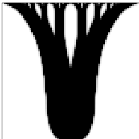
FIGURE 3.12 – Cas 3 avec critère d'arrêt sur f_0 et en entrée : n_x = n_y = 80 , \text{volfrac} = 0.4 , \text{penal} = 3 et \text{rmin} = 1.2
