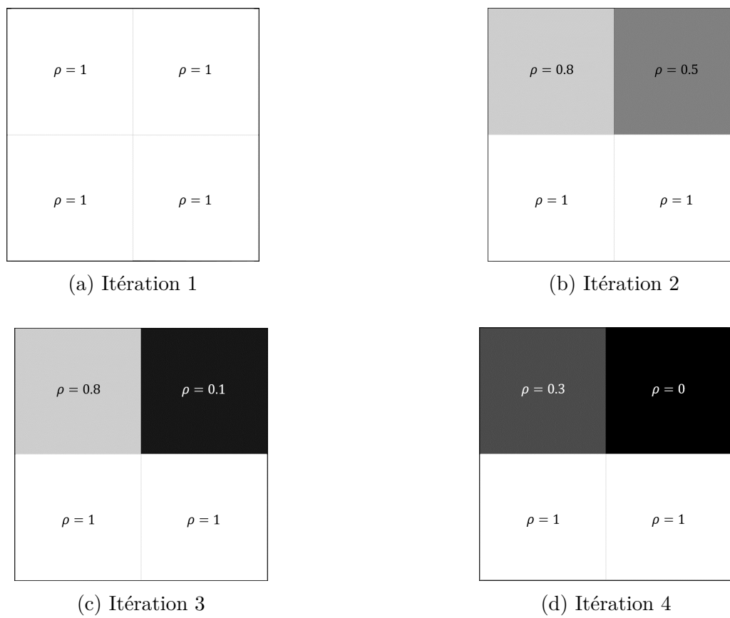
FIGURE 4.10 – Valeurs des variables de conception \rho_e du domaine 2x2 pour 4 itérations successives
