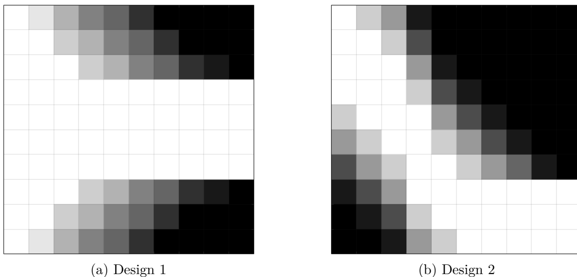
FIGURE 4.15 – Valeurs des variables de conception \rho_e du domaine 10x10 pour les deux designs considérés
