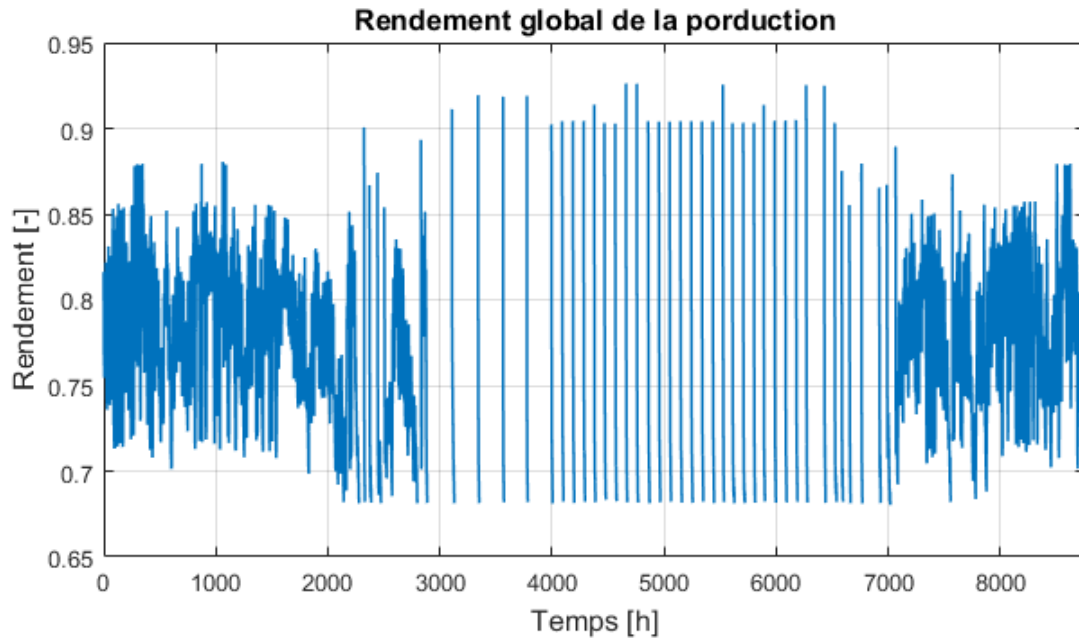
FIGURE 56 – Rendement de production d'énergie dans le cas où deux unités de cogénération par moteur Stirling et une chaudière d'appoint sont installés.
