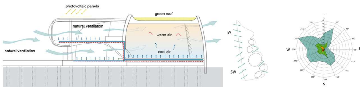
Figure 61 : Coupe de principe bioclimatique (gauche) - Vents dominants (droite) tiré de Transolar, 2012
