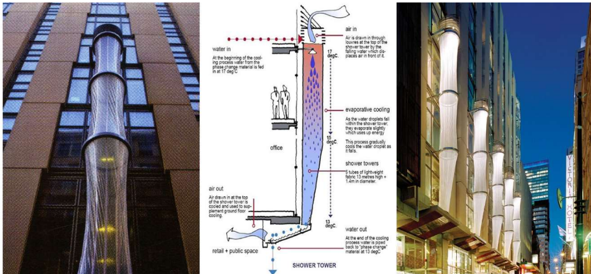
Figure 36 : CH2 - Fa ade Sud - Tours douches, tir  de DesignInc, 2013
