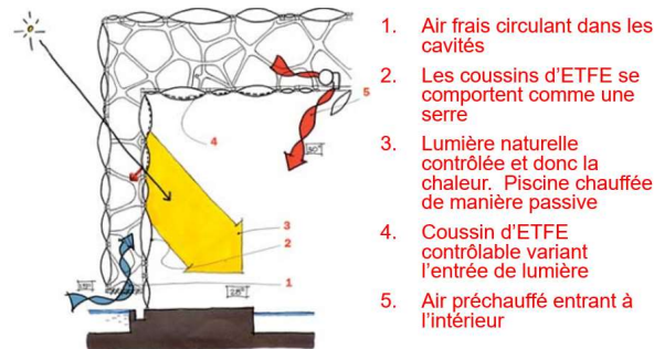
Figure 45 : Water Cube - Coupe de principe bioclimatique tiré de Gonchar, 2008, p.2
