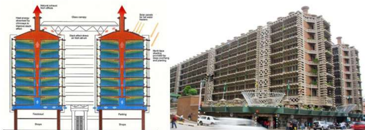
Figure 73 : Eastgate Center - Fonctionnement interne (EIDin & al., 2016)
