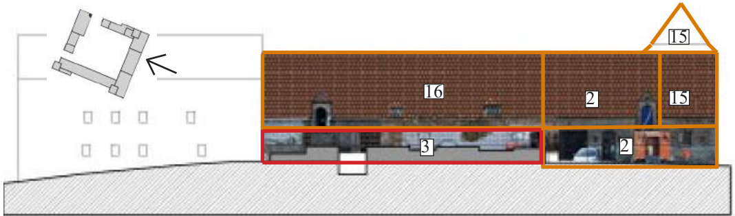
Élévation de l'aile est - Côté rue
