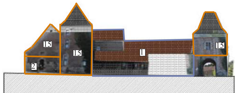
Élévation de l'aile nord - Côté rue
