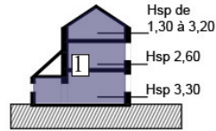
Coupe CC'
