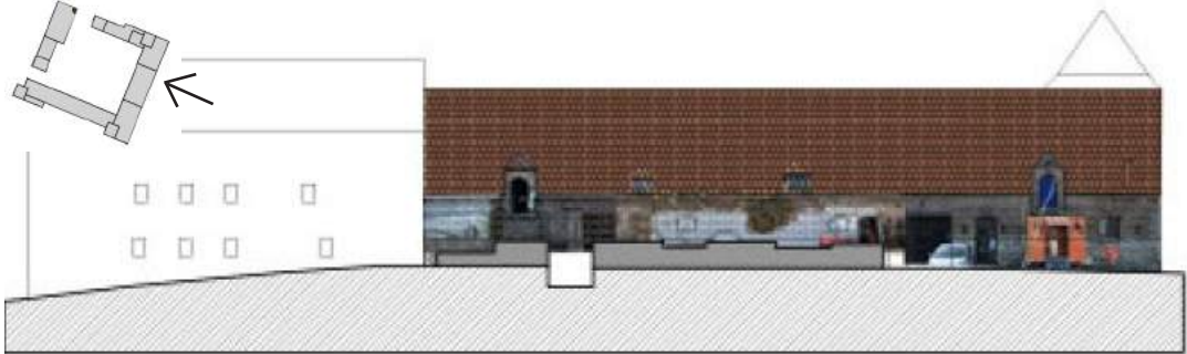
Élévation de l'aile est - Côté rue
