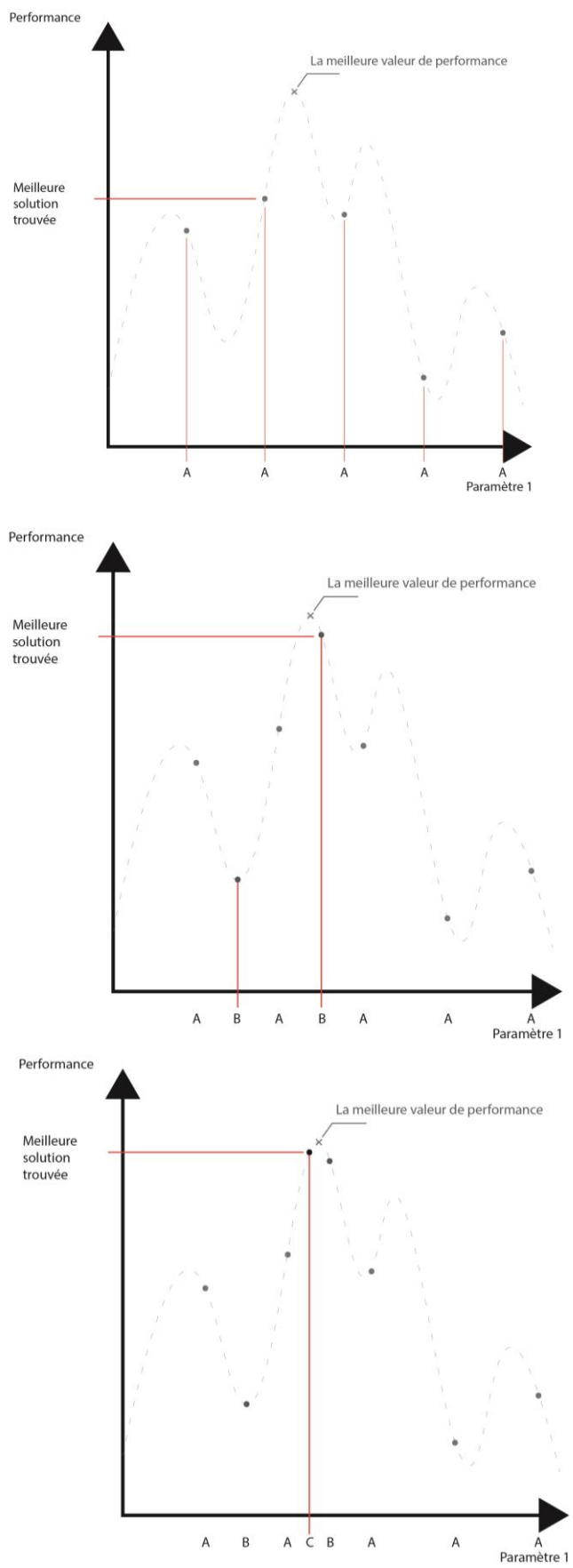
Fig. 17 : Exemple de recherche d'un optimum par recherche directe.
