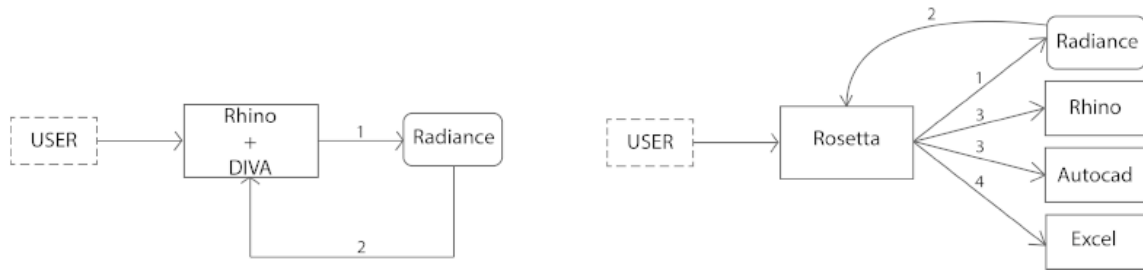
Fig.1 : Comparaison entre un workflow type et un workflow utilisant Rosetta [Leitao, 2017]
