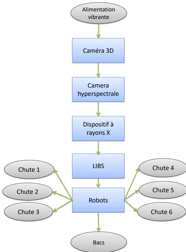
FIGURE 3.2 – Flux de matière du prototype Pick-It.
