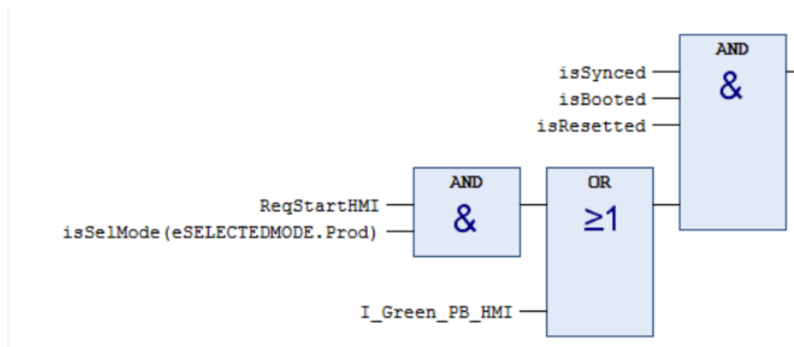
FIGURE 5.3 – Condition de transition pour le démarrage de la production écrit en Fonction Bloc Diagram avec TwinCAT3.
