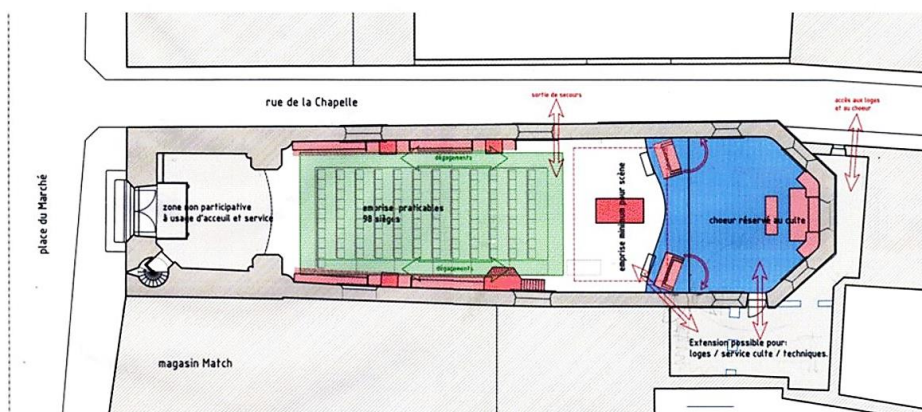
Figure 64 : Plan du projet
