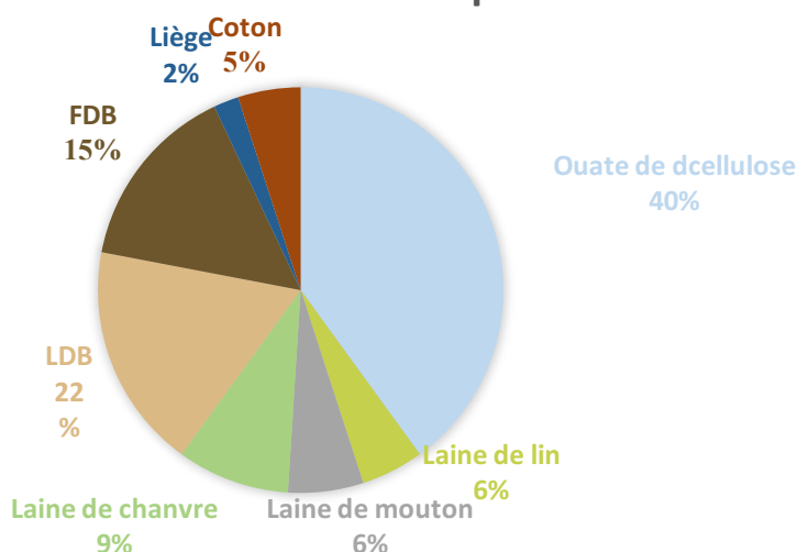
Graphique 7 : Estimation de la répartition des parts de marché de l'isolation biosourcée en France en 2014
