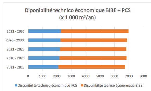
Graphique 13 : Cumul du volume de disponibilité technico-économique des PCS et BIBE entrant dans la fabrication des F-LDB en milliers de m 3 /an.
