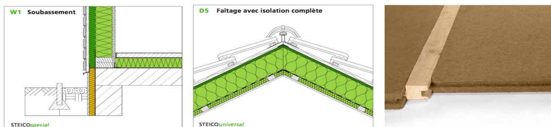
Illustration 4 : Procédé de mise en œuvre des FDB en ITE murale (à gauche), en pare-pluie pour toiture (au centre) et en système à lambourdes intégrées (à droite)
