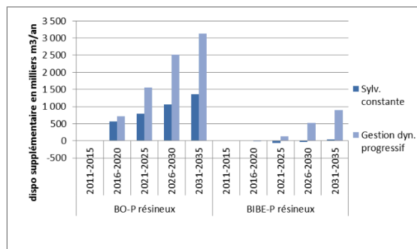
Graphique 12 : Volume de disponibilité nette supplémentaire du bois résineux total selon le rapport de L'ADEME en milliers de m 3 /an.
