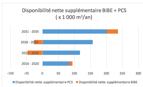
Graphique 14 : Cumul du volume de disponibilité nette supplémentaire des PCS et BIBE entrant dans la fabrication des F-LDB en milliers de m 3 /an.
