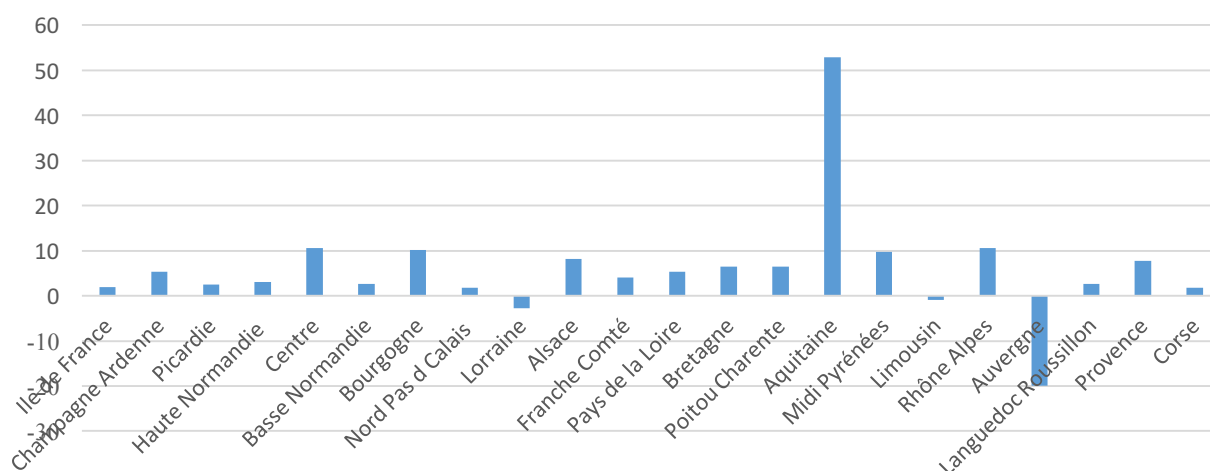
Graphique 16 : Cumul par régions des disponibilités nettes supplémentaires en BIBE et PCS résineux intégrés à la fabrication des F-LDB en milliers de m 3 /an.
