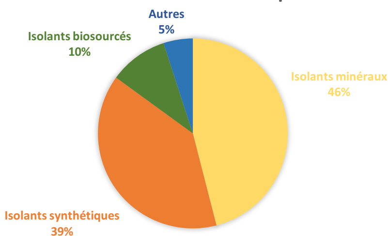
Graphique 6 : Estimation Répartition des parts de marché de l'isolation en France en 2017
