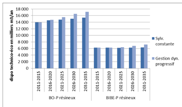
Graphique 11 : Volume de disponibilité technico-économique du bois résineux total selon le rapport de L'ADEME en milliers de m 3 /an.
