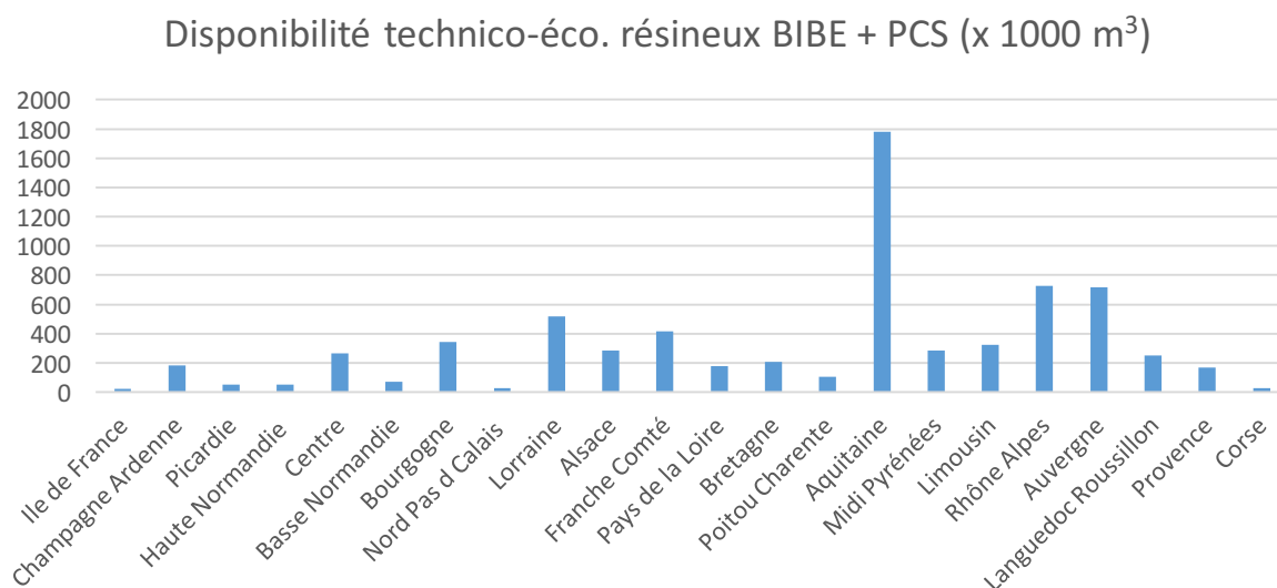
Graphique 15 : Cumul par régions des disponibilités technico-économiques en BIBE et PCS résineux intégrés à la fabrication des F-LDB en milliers de m 3 /an.
