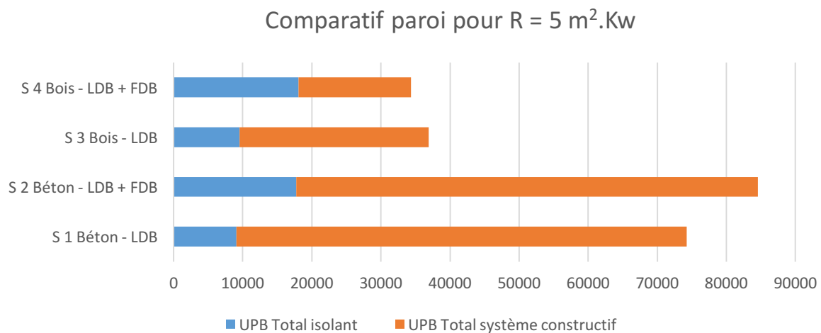
Graphique 22 : Mise en graphique de l'évaluation des Ecopoints UPB total des systèmes constructifs des 4 solutions
