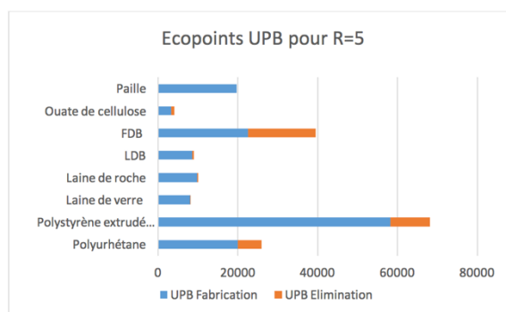
Graphique 21 : Mise en graphique du tableau 16 : Ecopoints UPB de matériaux isolants pour une UF de R = 5 \text{ m}^2 \cdot \text{K}/\text{W}
