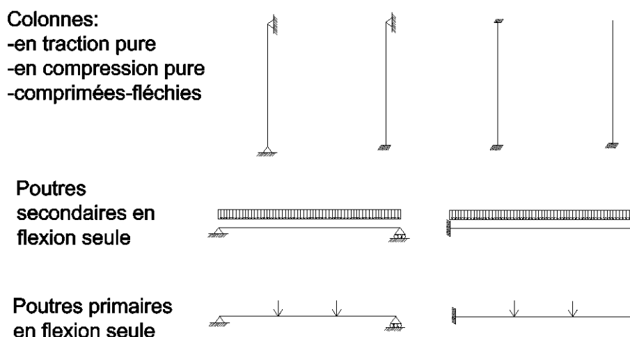
FIGURE 3.1 – Différents cas étudiés dans le cadre de l'étude locale de ce travail.
