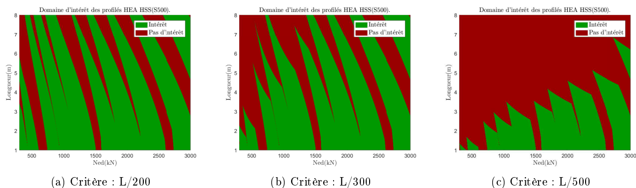
FIGURE 4.83 – Influence du critère de flèches sur l'intérêt des aciers HSS pour un élément comprimé-fléchi libre de flamber selon son axe fort mais empêché de déverser.
