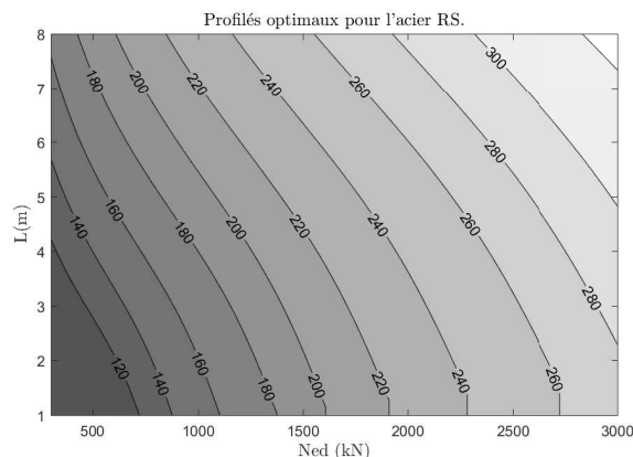
(b) Profils requis pour la nuance RS (S355)
