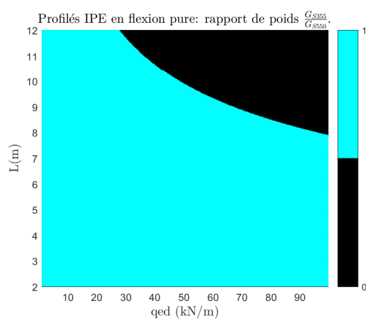
(b) Profils IPE S550 sans déversement
