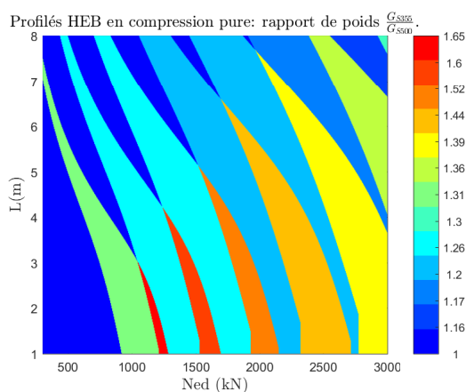
(a) Profils HEB S500
