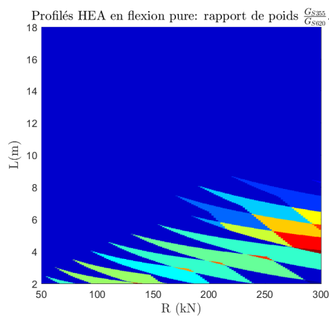
(c) Profilés HEA S620 avec déversement
