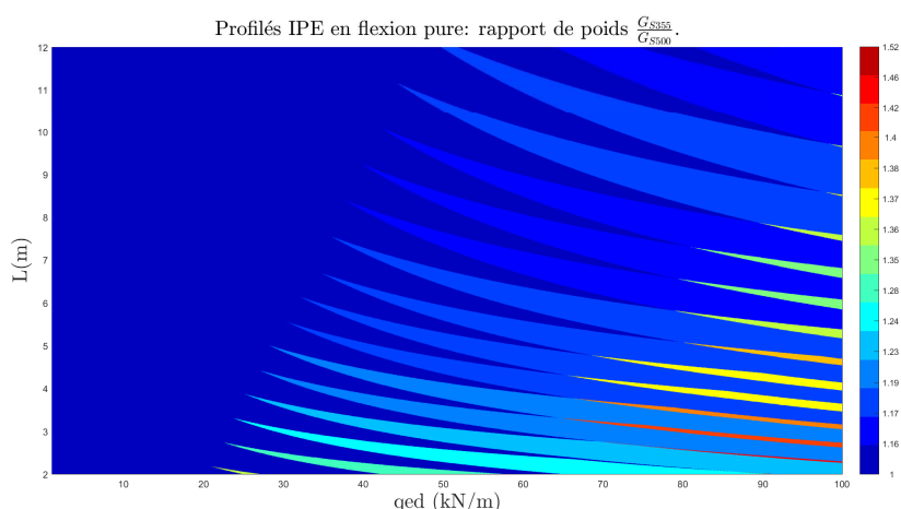
FIGURE 5.8 – Rapport de poids entre les profilés requis pour les deux nuances comparées pour une poutre secondaire bi-encastrée empêchée de déverser.
