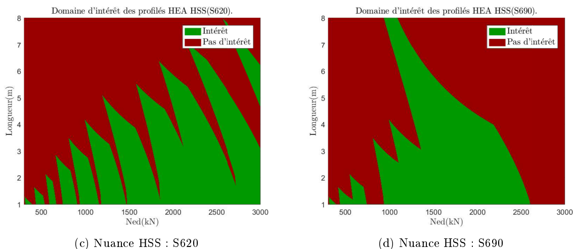
FIGURE 4.82 – Influence du choix de la nuance HSS sur l'intérêt de leur utilisation pour un élément comprimé-fléchi.
