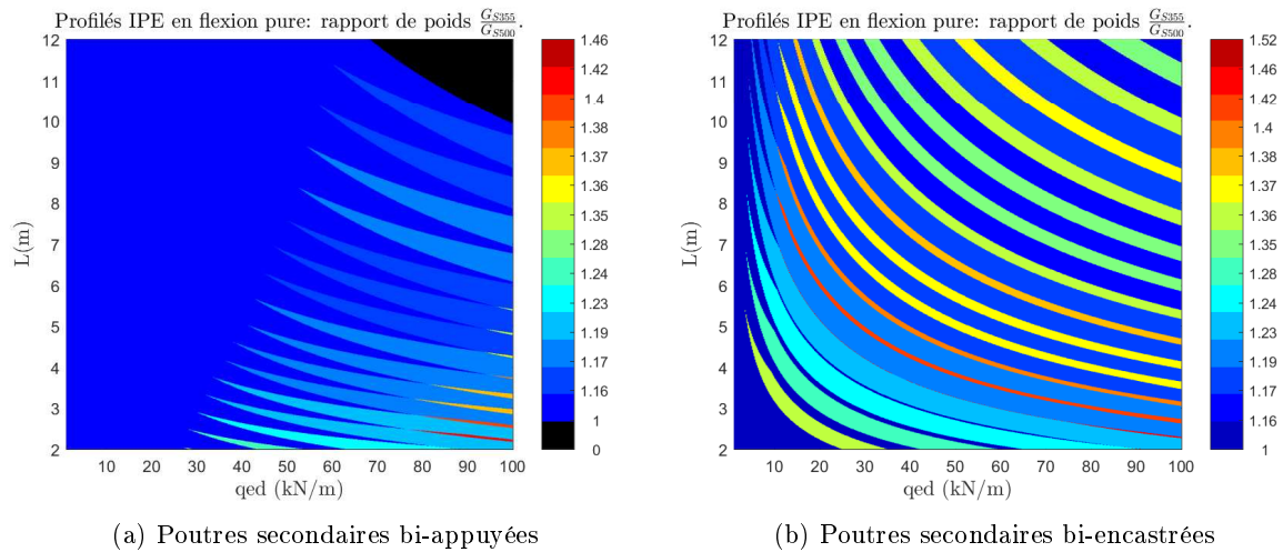
FIGURE 5.18 – Rapport de poids entre les deux profils requis pour des poutres secondaires bi-appuyées ou bi-encastrées sans déversement et cintrée initialement.
