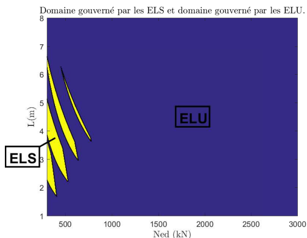
(b) Domaines gouvernés par les ELU-ELS
