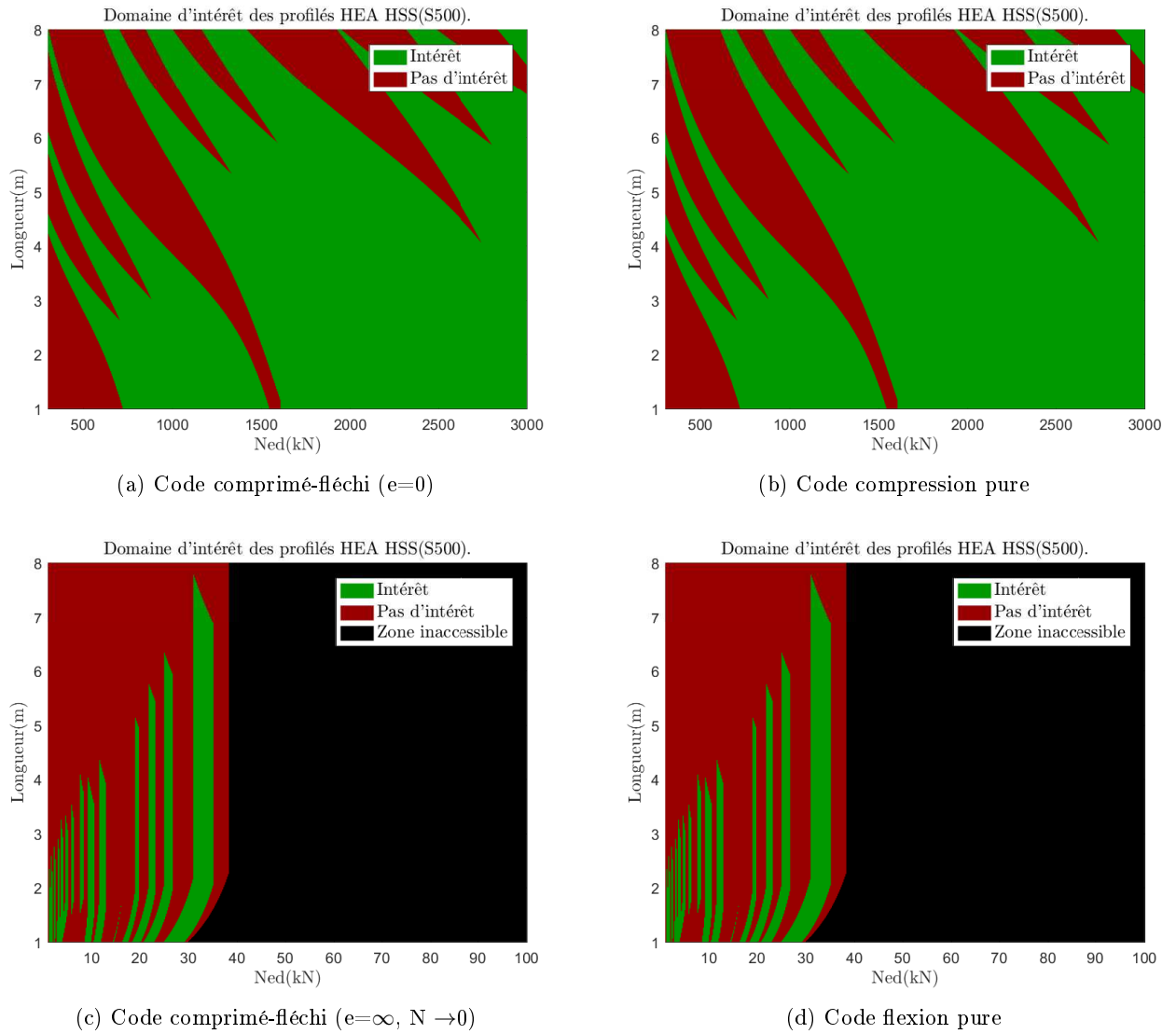
FIGURE 4.71 – Confrontation des résultats aux conditions limites pour le cas du flambement dans le plan sans déversement.
