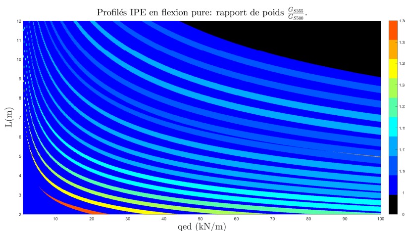
FIGURE 5.10 – Rapport de poids entre les profils requis pour les deux nuances comparées pour une poutre secondaire bi-encastée libre de déverser.
