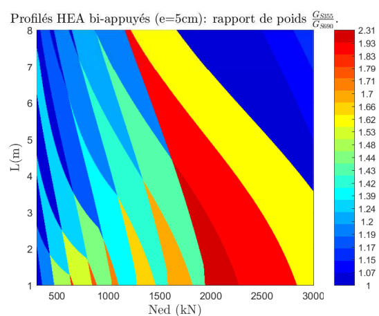
(d) HEA, bi-appuyés, e=5cm, S690
