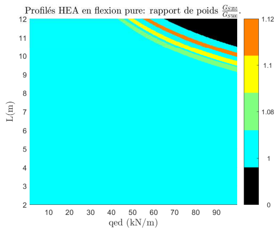
(a) Profils HEA S500 avec déversement
