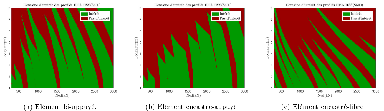
FIGURE 4.86 – Influence des conditions d'appuis sur les résultats pour un élément comprimé-fléchi avec flambement dans le plan sans déversement.
