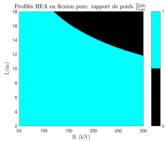
(d) Profils HEA S690 avec déversement
