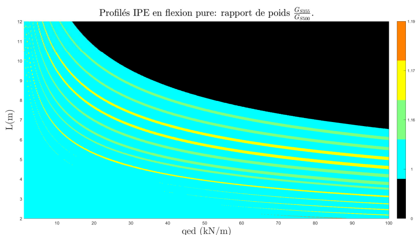
FIGURE 5.7 – Rapport de poids entre les profilés requis pour les deux nuances comparées pour une poutre secondaire bi-appuyée libre de déverser.
