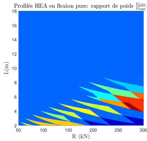
(a) Profilés HEA S500 avec déversement
