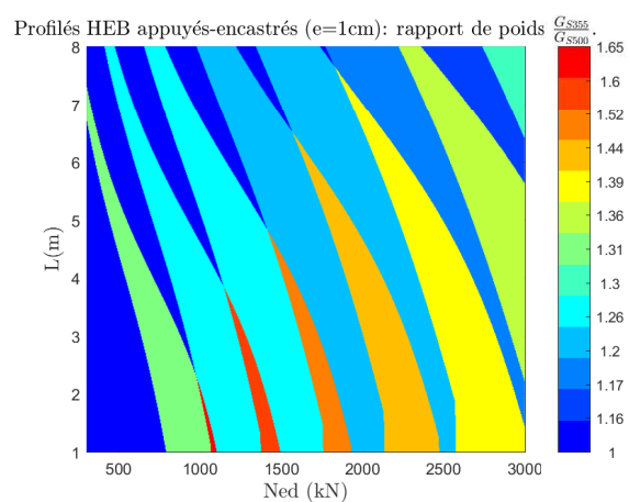
(a) HEB, appuyés-encastrés, e=1cm, S500
