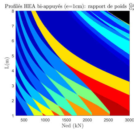
(d) HEA, bi-appuyés, e=1\text{cm} , S690
