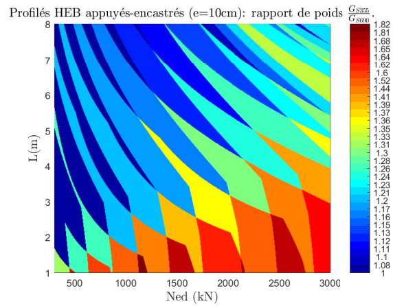
(d) HEB, appuyés-encastres, e=10\text{cm} , S690
