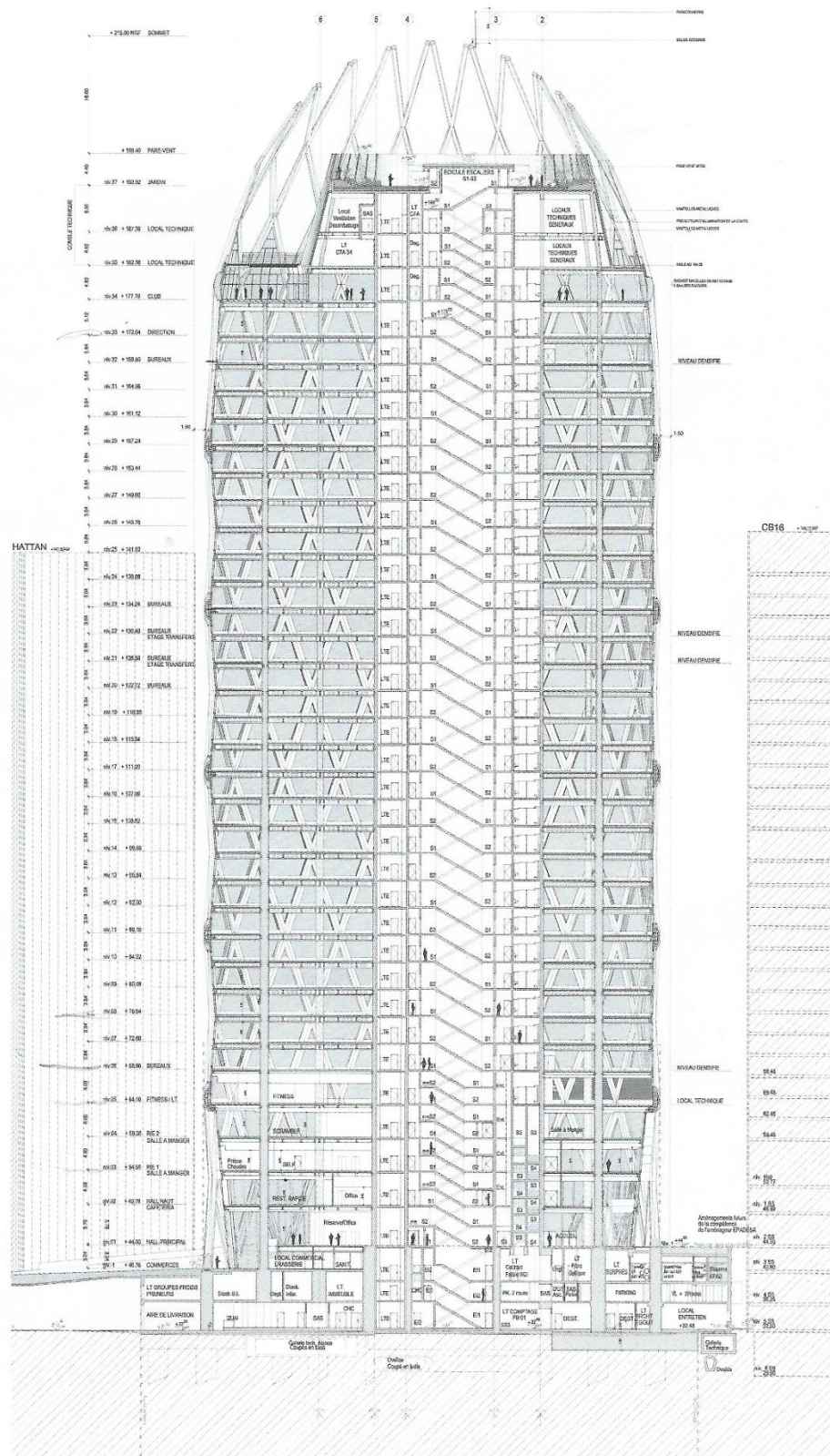
Figure 2 Tour D2 - coupe longitudinale
