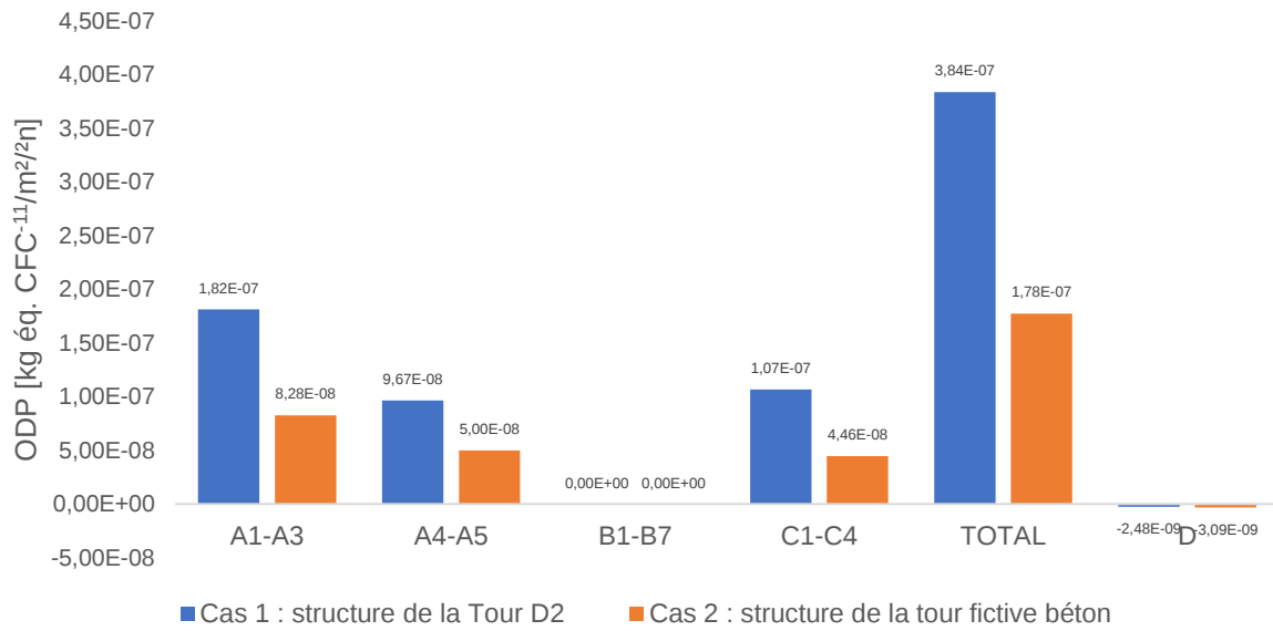
Figure 27 : Comparaison ODP
