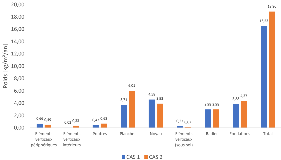
Figure 2 : Comparaison du poids des structures
