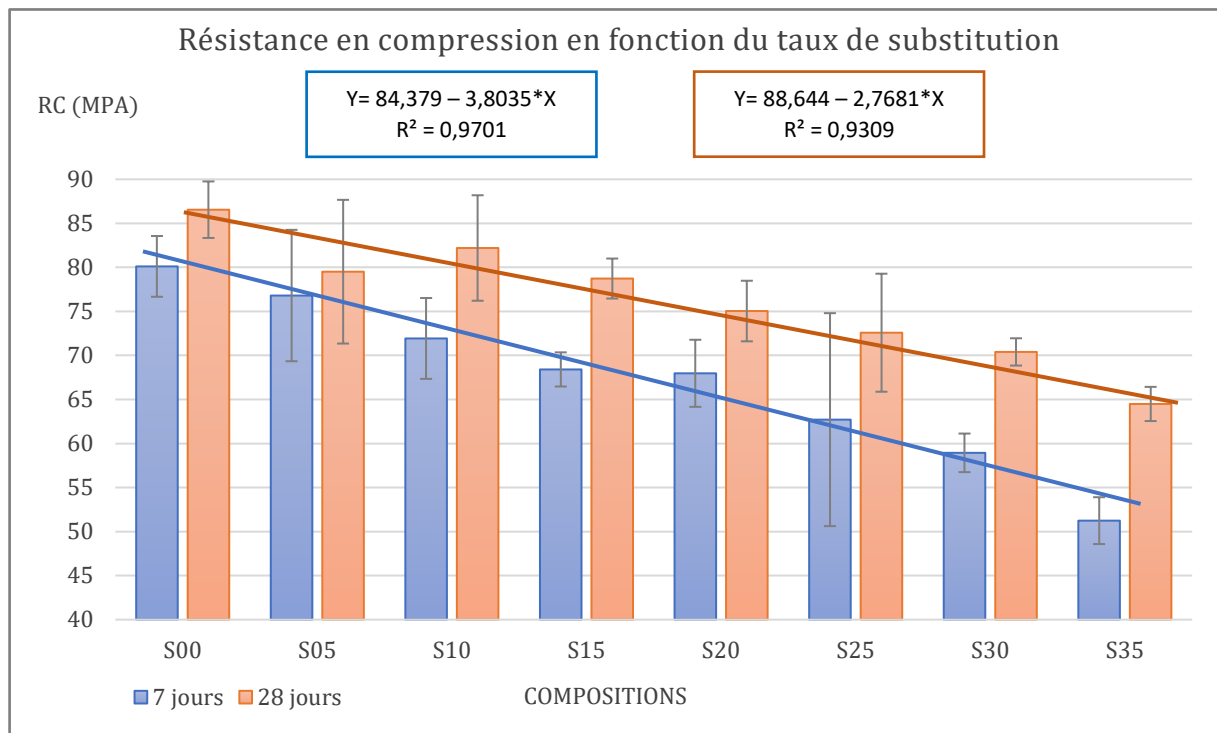
Figure 5: Évolution de la résistance en compression en fonction du taux de substitution.
